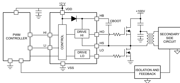
典型应用图
