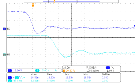
C_L = 1\text{nF} V_{DD} = 12\text{V} 图 7-6. HO 下降时间和 HI 至 HO 关断传播延迟
