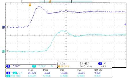
C_L = 1\text{nF} V_{DD} = 12\text{V} 图 7-5. HO 上升时间和 HI 至 HO 导通传播延迟
