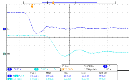
图 7-6. HO 下降时间和 HI 至 HO 关断传播延迟
