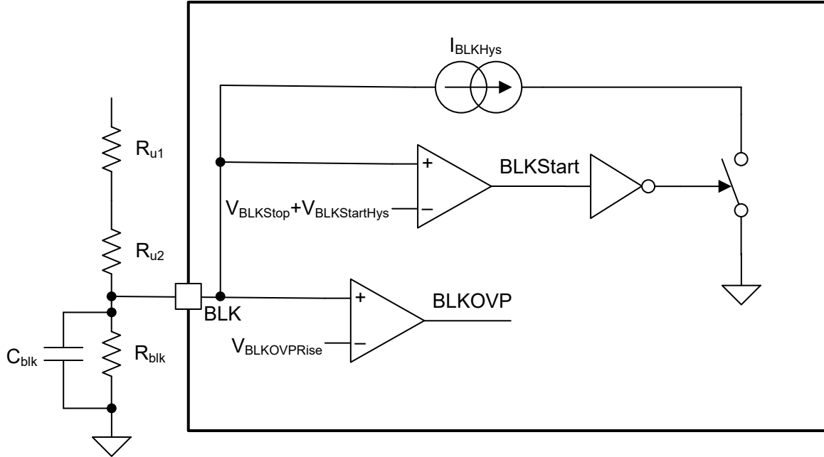
图 7-7. BLK 引脚输入电压检测架构
