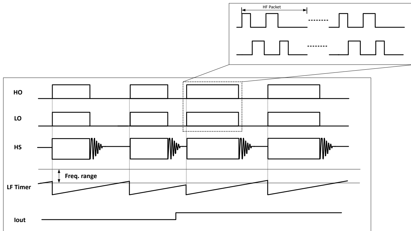
图 7-19. LF 突发中的包大小调节
