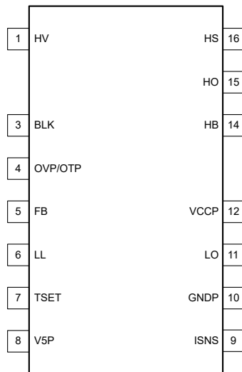
图 5-1. DDB 封装，16 引脚 SOIC；移除了引脚 2 和 13 (顶视图)
