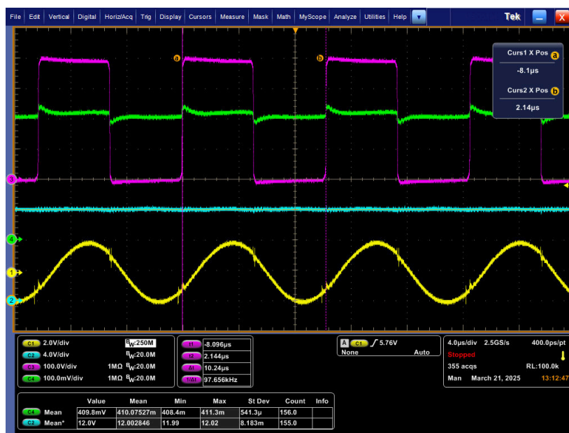
图 8-4. 15A 负载、390V 输入时的稳定状态波形 ( Ch1 = ISNS ; Ch2 = Vout ; Ch3 = SW ; Ch4 = I_OPT )
