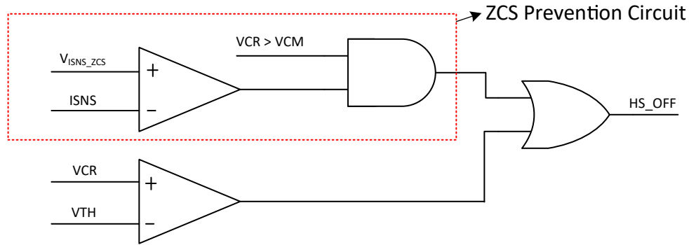
图 7-10. 高侧 MOSFET 导通时的 ZCS 预防方案
