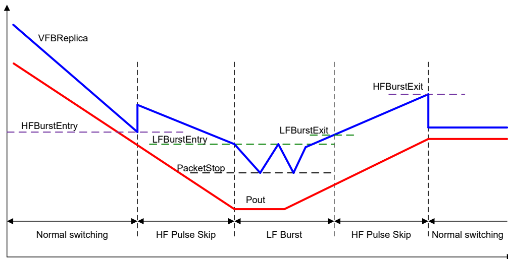
图 7-20. 通过 FBReplica 比较器确定突发模式
