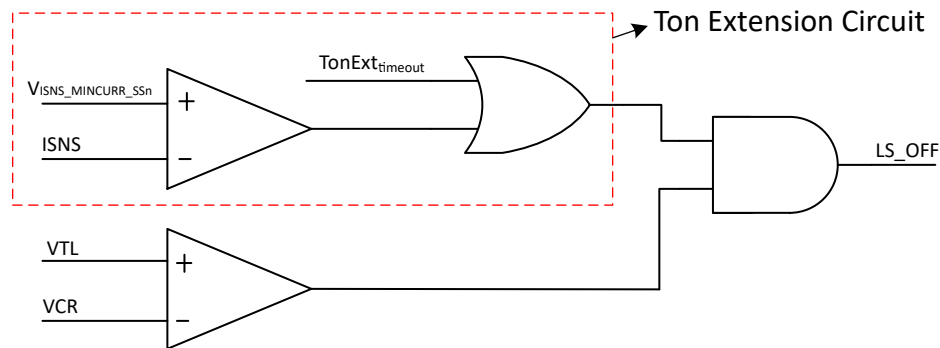
图 7-11. Ton 延长方案
