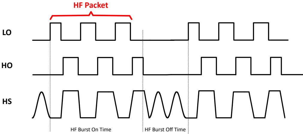
图 7-17. 高频脉冲跳跃包
