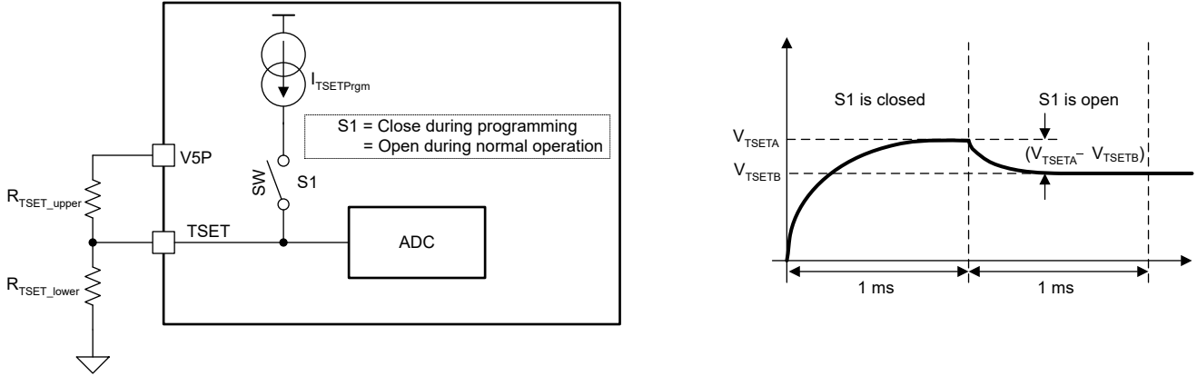
图 7-4. TSET 引脚编程
