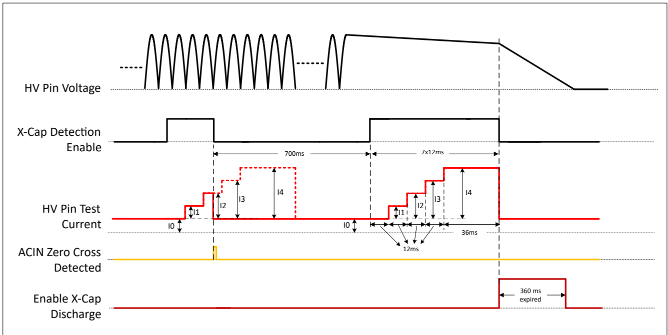
图 7-22. 过零检测序列仅 HV 引脚
