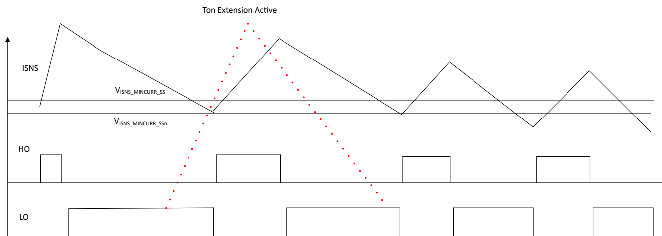
图 7-12. 启动期间的 ZCS 预防
