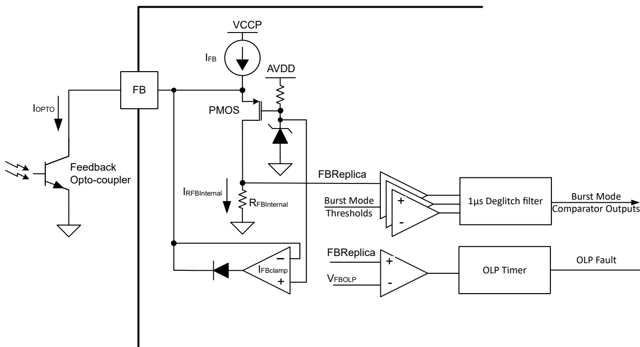
图 7-5. 反馈链方框图
