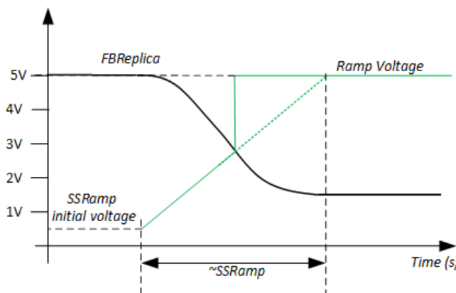
图 7-16. 软启动运行
