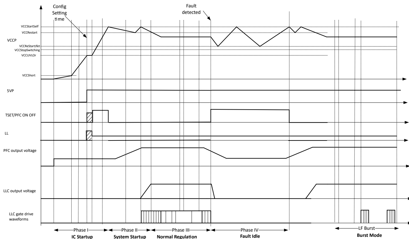
图 7-14. 启用“HV 启动”功能时的启动顺序
