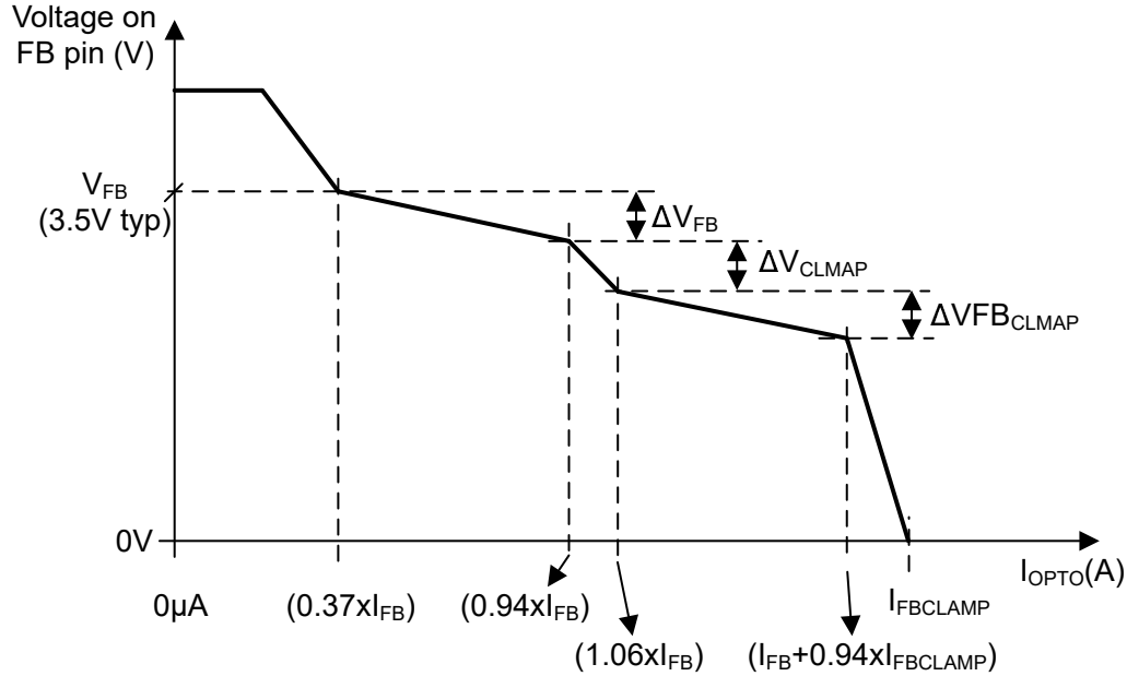
图 7-6. FB 引脚电压与 FB 引脚电流间的关系
