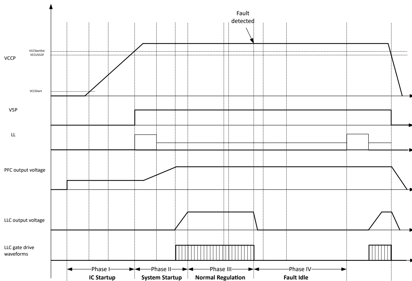
图 7-15. 禁用“HV 启动”功能时的启动顺序
