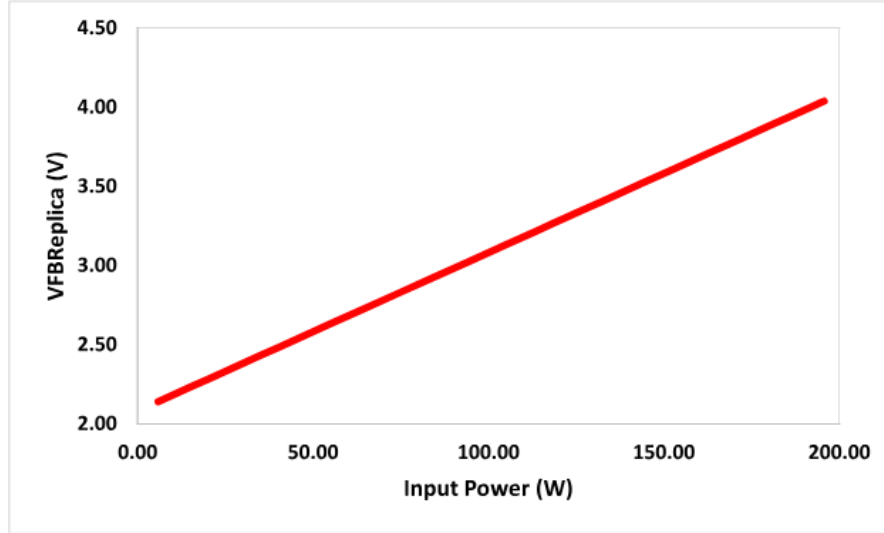
图 8-2. FBReplica 与 P_{in} 间的关系
