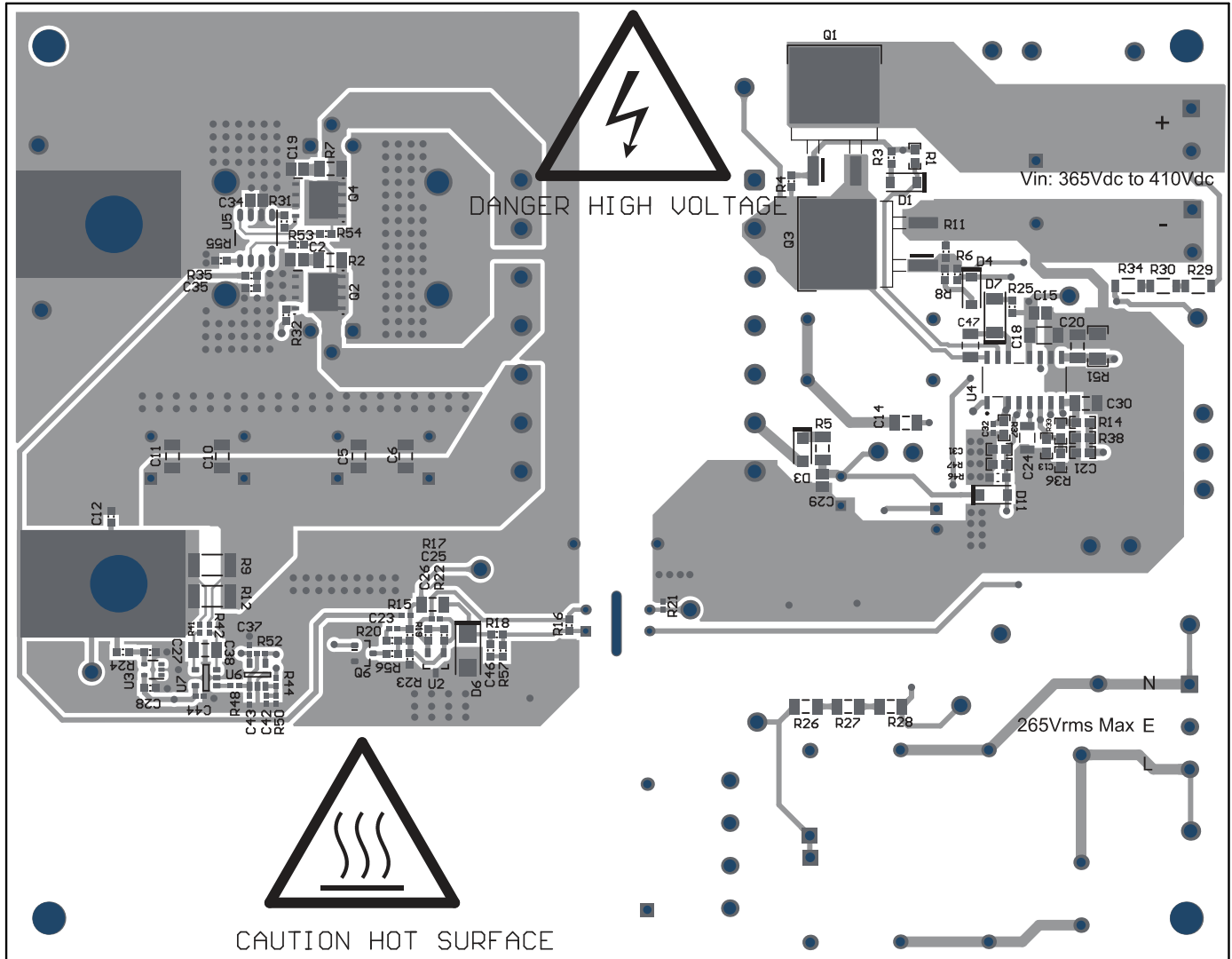
图 8-8. UCC25661EVM-128 (底视图)
