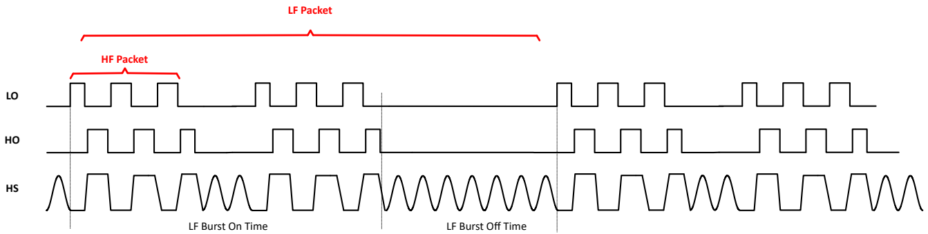
图 7-18. 低频突发包
