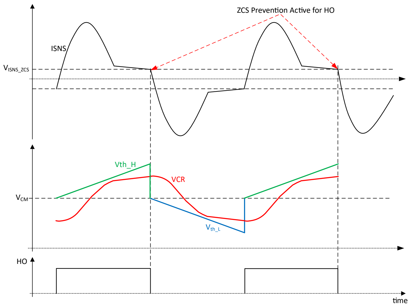
图 7-9. ZCS 保护
