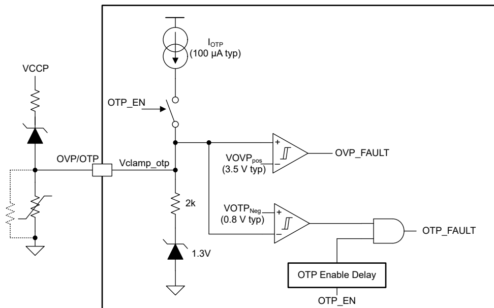
图 7-8. OVP/OTP 保护架构
