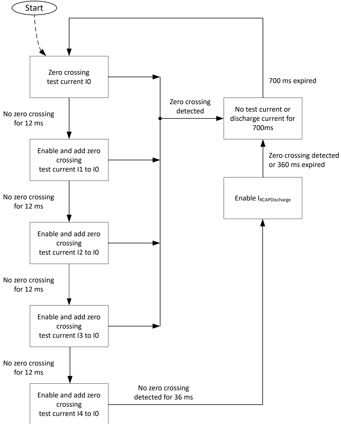
图 7-23. 交流 ZCD 和 X 电容器放电流程图
