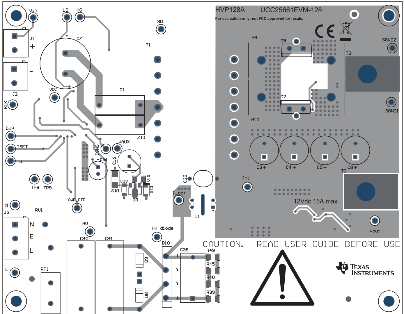
图 8-7. UCC25661EVM-128 ( 顶视图 )
