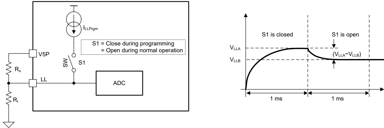
图 7-21. LL 引脚编程
