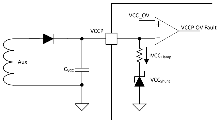
图 7-13. VCC 钳位
