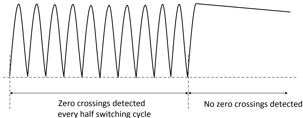
图 44. 交流电断开波形
