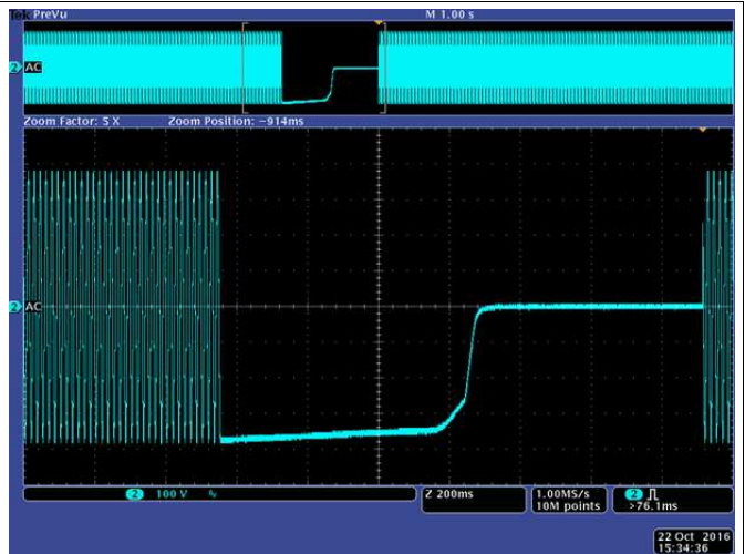
图 61. X 电容器放电
