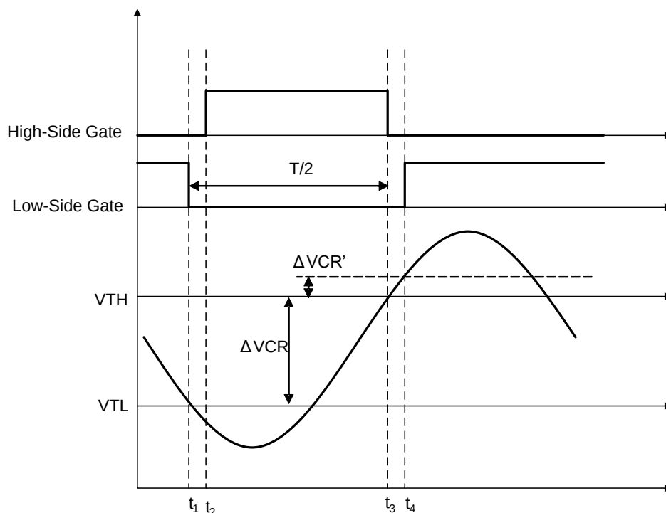
图 29. HHC 栅极打开/关闭控制原则
