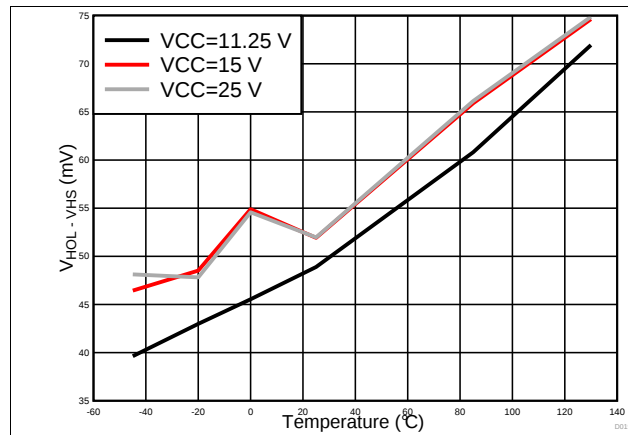
图 19. V_{\text{HOL}} - V_{\text{HS}} 与温度间的关系
