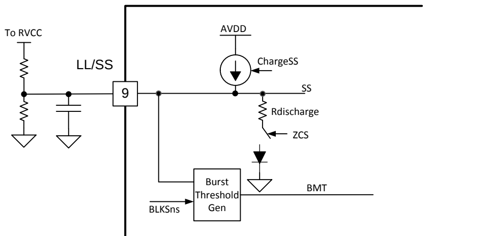
图 37. LL/SS 方框图
