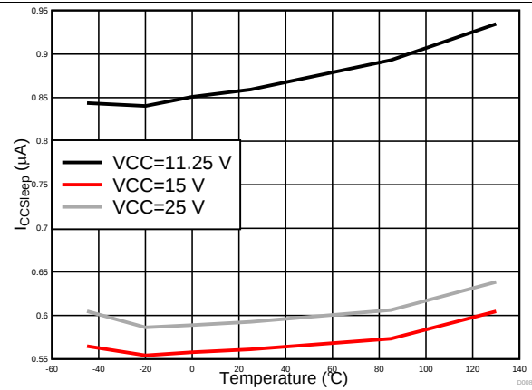
图 8. I_{CCSleep} 与温度间的关系
