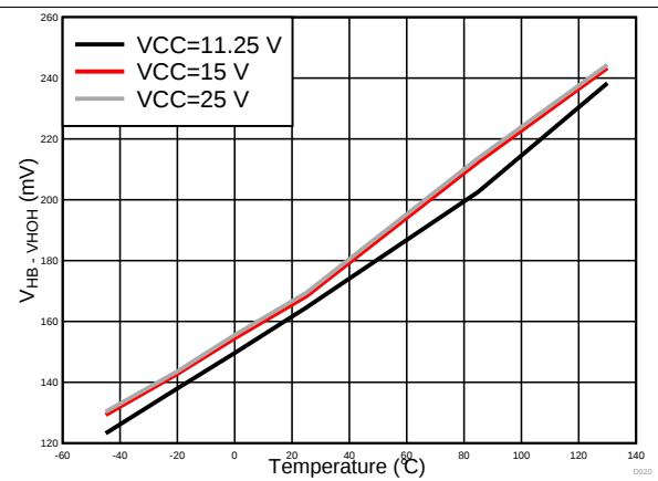
图 20. V_{\text{HB}} - V_{\text{HOH}} 与温度间的关系
