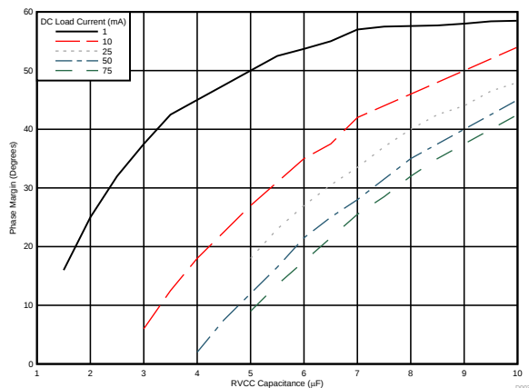
图 51. RVCC 引脚电容器
