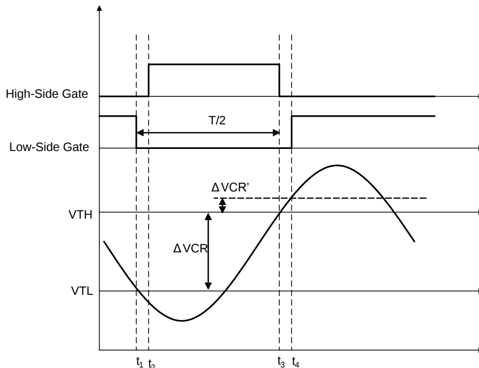
图 22. HHC 栅极打开/关闭控制原则
