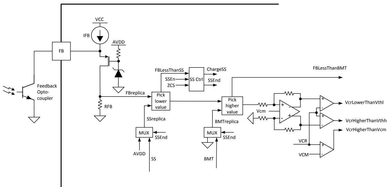
图 23. 反馈链方框图
