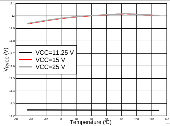
图 7. V_{RVCC} 与温度间的关系, I_{CC} = 0\text{mA}
