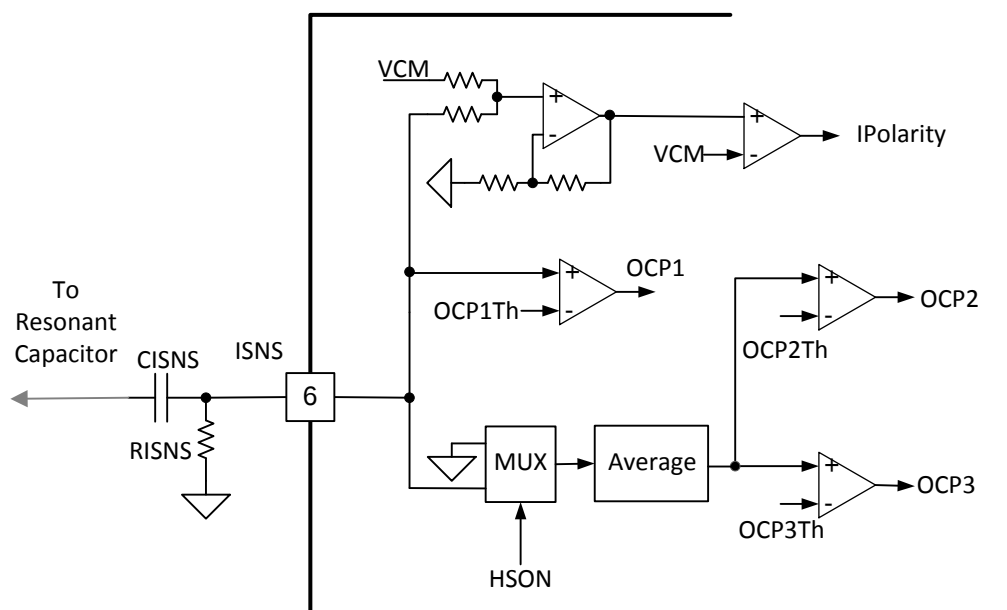
图 28. ISNS 方框图
