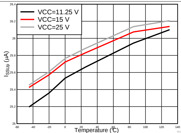
图 13. I_{SSUP} 与温度间的关系
