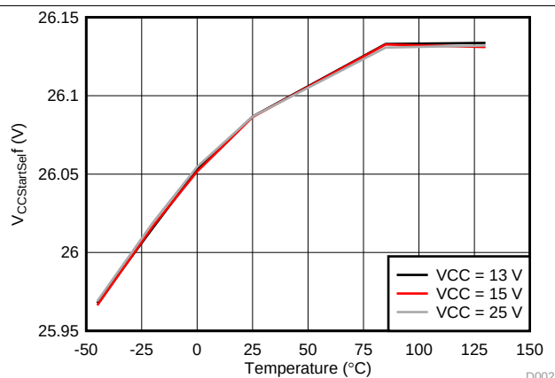
图 26. V_{CCStartSelf} 与温度间的关系
