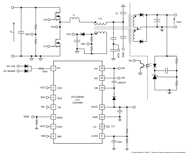
简化原理图
