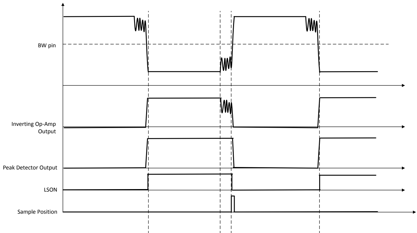
图 39. BW 感应块时序图
