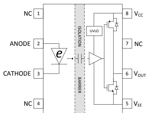
UCC23514V 的功能方框图
