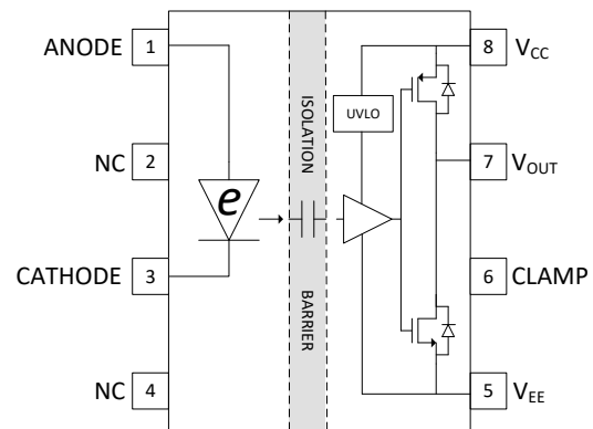
UCC23514M 的功能方框图
