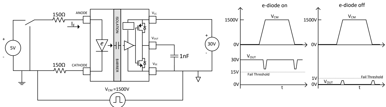
图 7-3. CMTI Test Circuit
