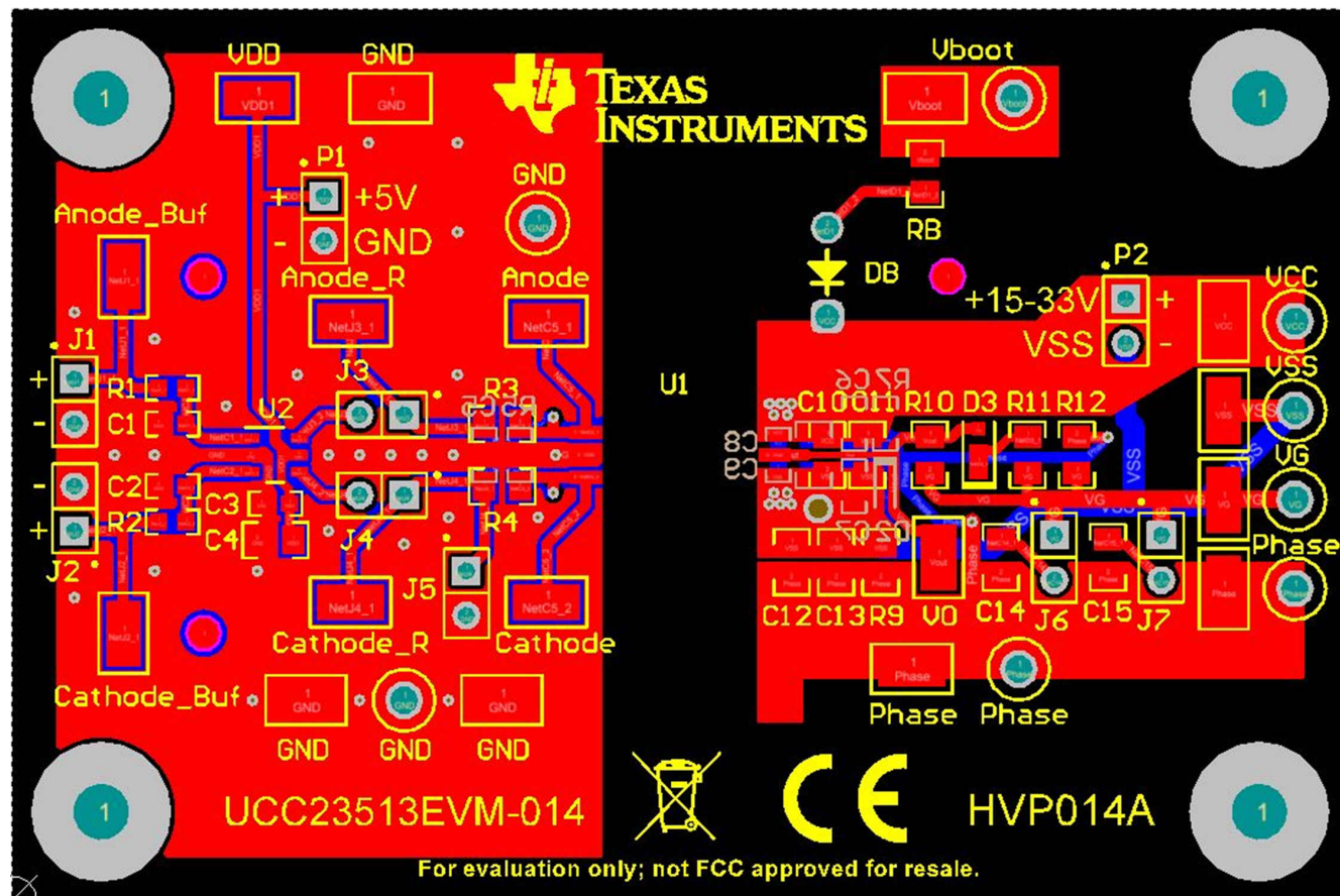
图 12-1. Layout Example
