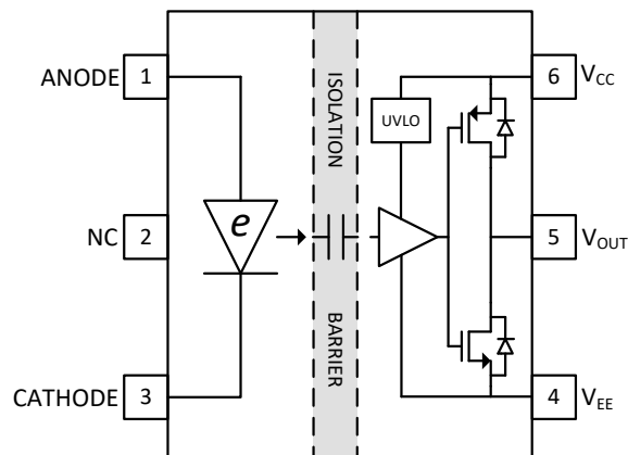
UCC23511-Q1 (SO6) 的功能方框图
