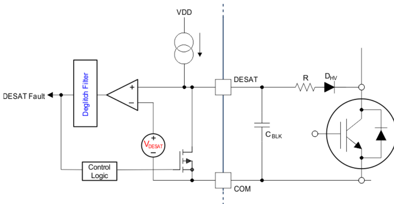
图 7-5. DESAT Protection
