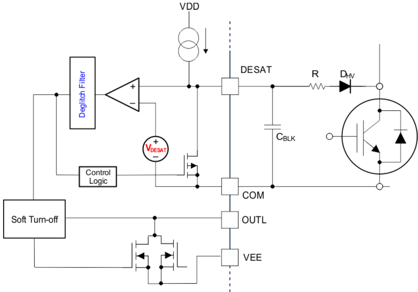
图 7-6. Soft Turn-off
