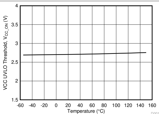
图 5-11. VCC UVLO vs Temperature
