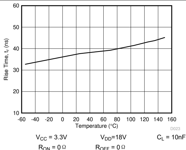
图 6-16. t_r Rise Time vs Temperature
