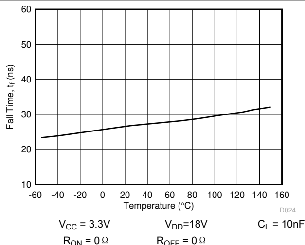
图 6-17. t_f Fall Time vs Temperature
