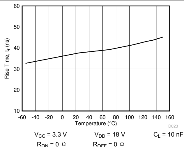
图 6-16. t_r Rise Time vs Temperature
