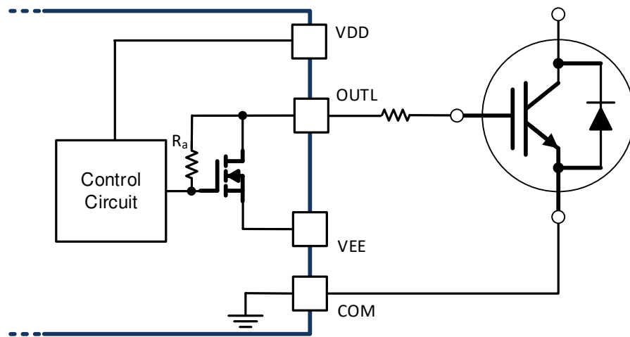
图 8-2. Active Pulldown
