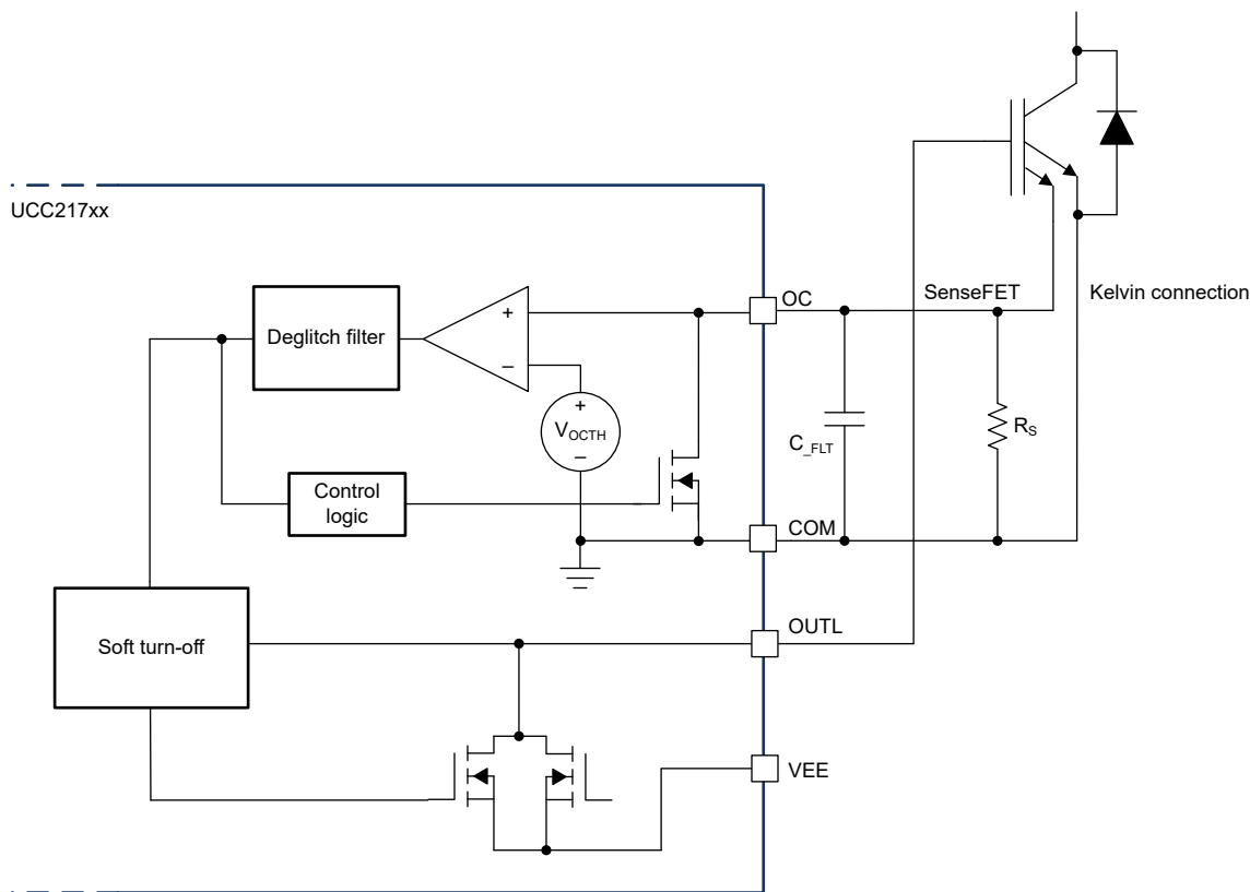
图 8-6. Soft Turn-off
