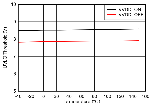
图 5-23. VDD 8V UVLO 阈值与温度之间的关系
