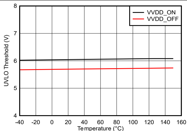
图 5-21. VDD 5V UVLO 阈值与温度间的关系
