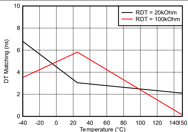
图 5-31. 死区时间匹配与温度之间的关系 ( R_{DT} = 20\text{k}\Omega 和 100\text{k}\Omega )
