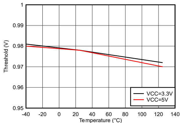
图 5-28. IN/EN 低阈值
