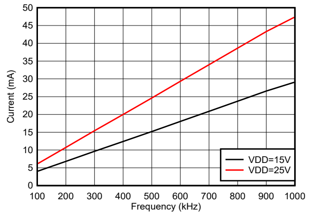
图 5-7. 每通道电流消耗 ( I_{VDDA/B} ) 与频率之间的关系 (1nF 负载, V_{DD} = 15V 或 25V )
