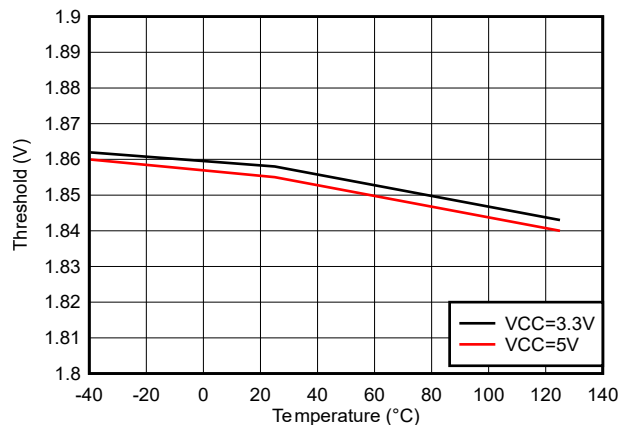
图 5-29. IN/EN 高阈值
