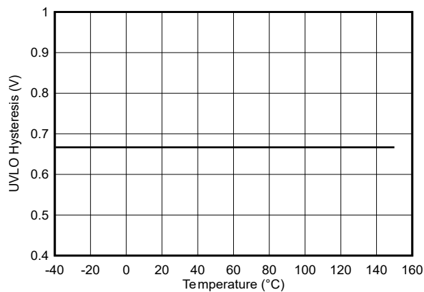
图 5-22. VDD 8V UVLO 迟滞与温度之间的关系
