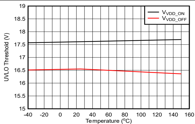
图 5-25. VDD 17-V UVLO 阈值与温度之间的关系
