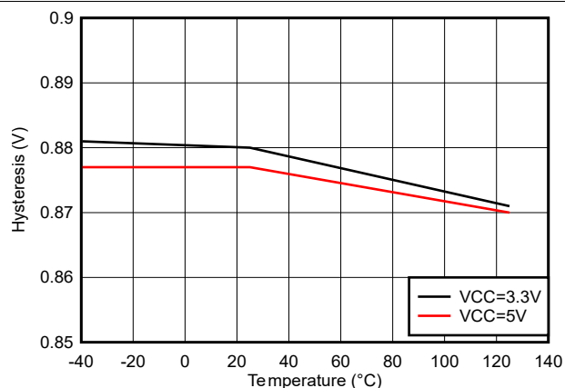
图 5-27. IN/EN 迟滞与温度之间的关系
