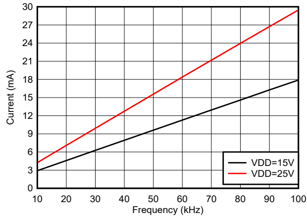
图 5-8. 每通道电流消耗 ( I_{VDDA/B} ) 与频率之间的关系 (10nF 负载, V_{DD} = 15V 或 25V )
