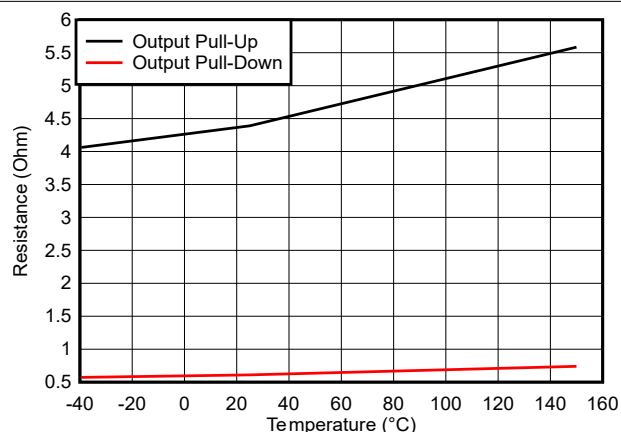
图 5-13. 输出电阻与温度之间的关系
