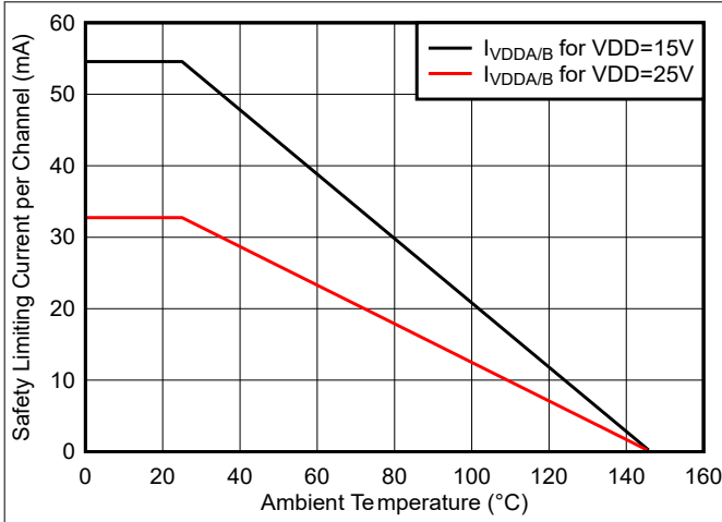
图 5-1. 根据 VDE 标准 DWK 封装限制电流的热降额曲线 (两个通道同时运行时每个通道的电流)
