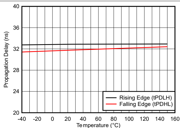
图 5-14. 传播延迟与温度间的关系
