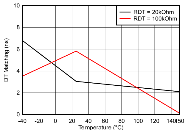
图 5-29. 死区时间匹配与温度之间的关系 ( R_{DT} = 20\text{k}\Omega 和 100\text{k}\Omega )
