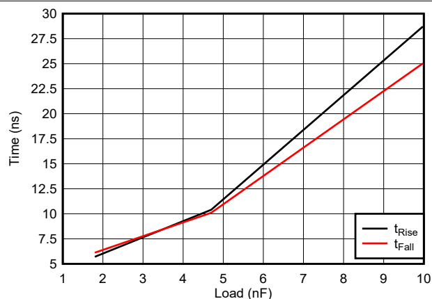
图 5-12. 上升和下降时间与负载间的关系 (VDD = 15V)
