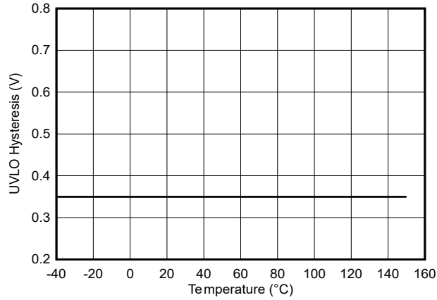
图 5-20. VDD 5V UVLO 迟滞与温度间的关系
