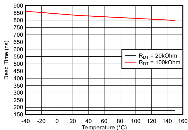
图 5-28. 死区时间与温度之间的关系 ( R_{DT} = 20\text{k}\Omega 和 100\text{k}\Omega )
