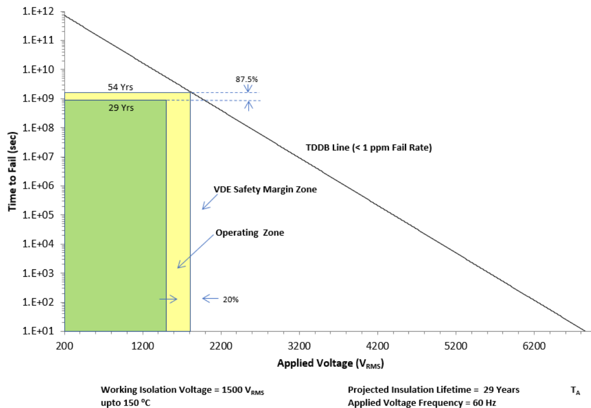
图 5-5. 增强型隔离电容器寿命预测
