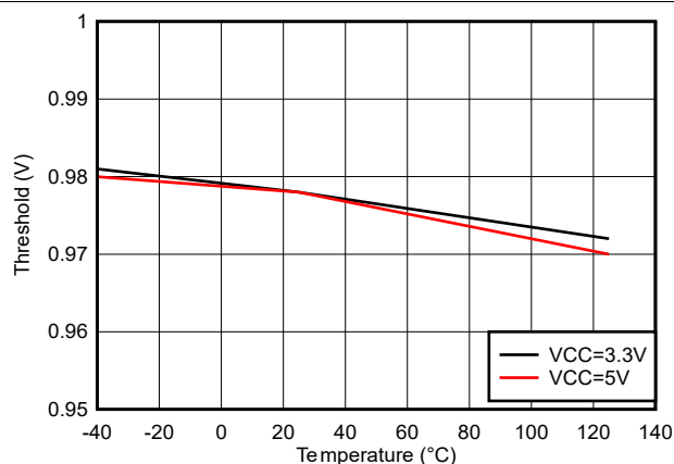
图 5-26. IN/DIS 低阈值
