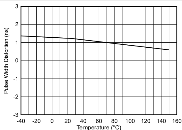
图 5-16. 脉宽失真度与温度之间的关系
