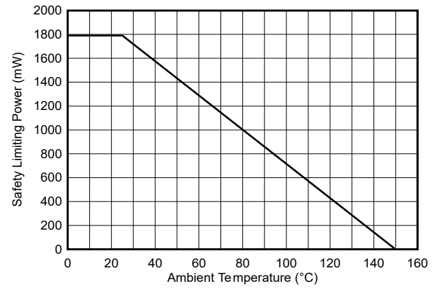
图 5-4. 根据 VDE 标准 DW 封装安全相关限制功率的热降额曲线
