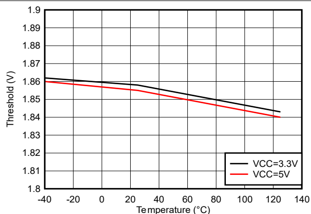
图 5-27. IN/DIS 高阈值
