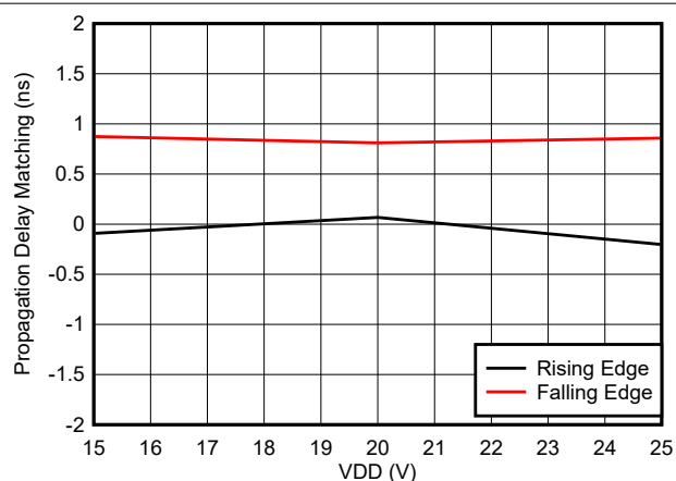
图 5-17. 传播延迟匹配 ( t_{\text{DM}} ) 与 VDD 之间的关系
