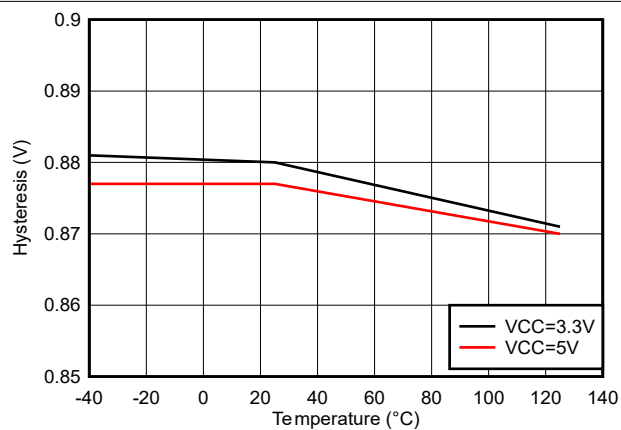
图 5-25. IN/DIS 迟滞与温度之间的关系
