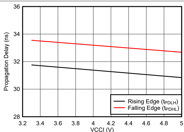
图 5-15. 传播延迟与 VCCI 之间的关系
