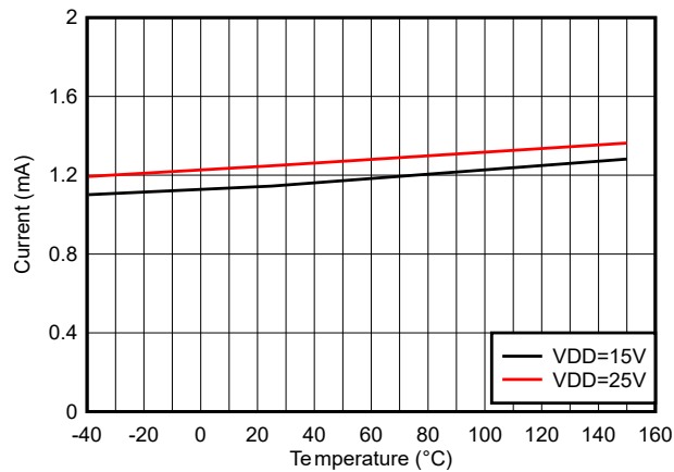
图 5-10. 每通道 ( I_{VDDA/B} ) 静态电源电流与温度之间的关系 (无负载, 低电平输入, 无开关)
