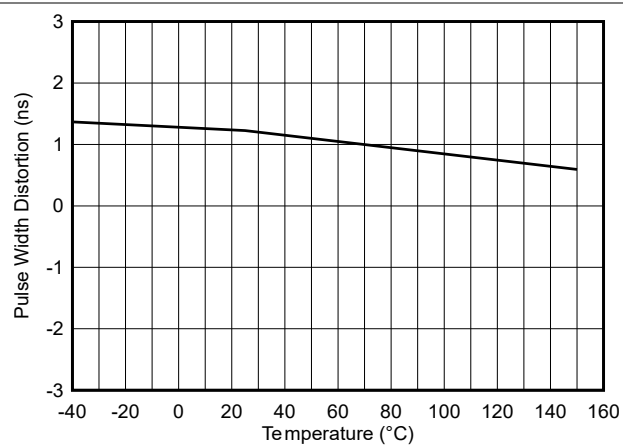
图 6-16. 脉宽失真度
