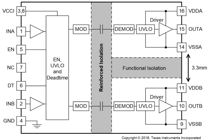
功能方框图
