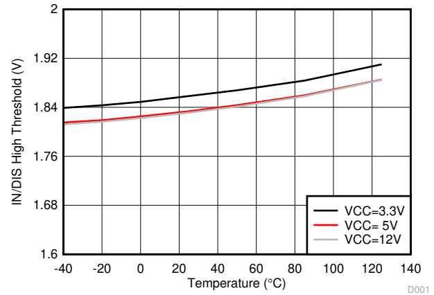
图 5-23. INA/B/EN 高阈值
