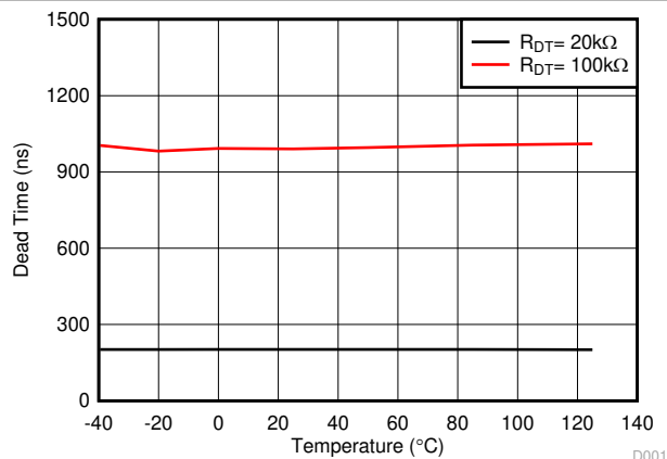
图 5-24. 死区时间与温度之间的关系 ( R_{DT} = 20\text{k}\Omega 和 100\text{k}\Omega )
