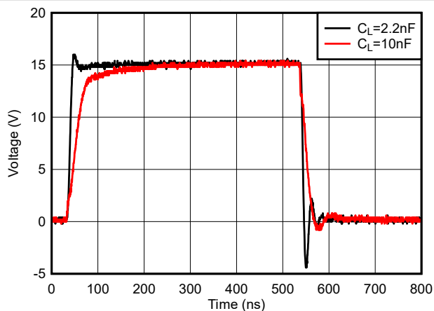
图 5-26. 典型输出波形
