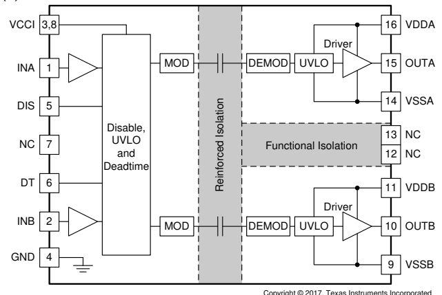
功能方框图
