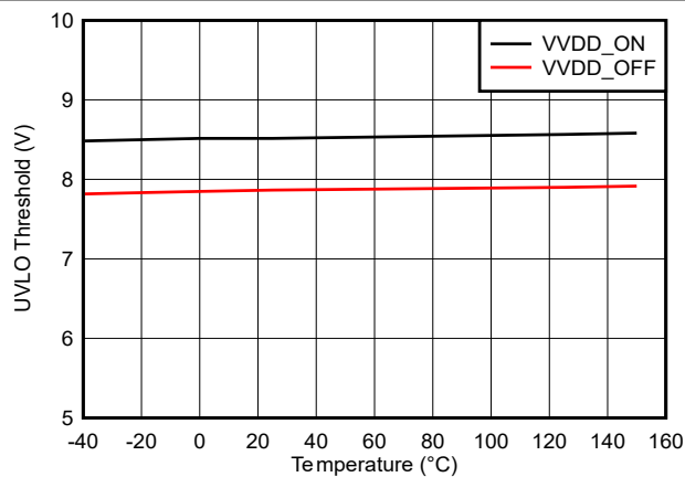
图 5-20. VDD 8V UVLO 阈值与温度之间的关系
