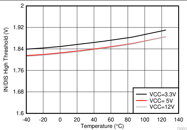
图 5-23. IN/DIS 高阈值
