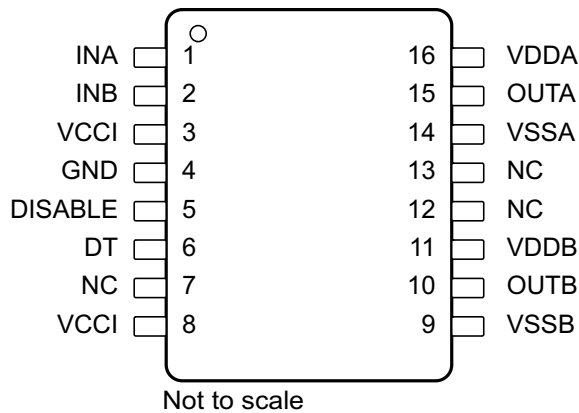
图 4-1. DW 封装 16 引脚 SOIC 顶视图
