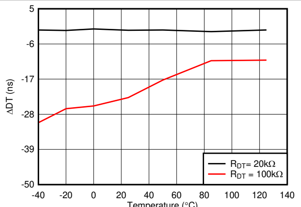
图 5-25. 死区时间匹配与温度之间的关系 ( R_{DT} = 20\text{k}\Omega 和 100\text{k}\Omega )
