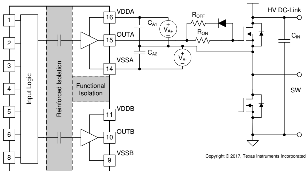
图 8-3. 利用两个 LSO 偏置电源生成负偏置
