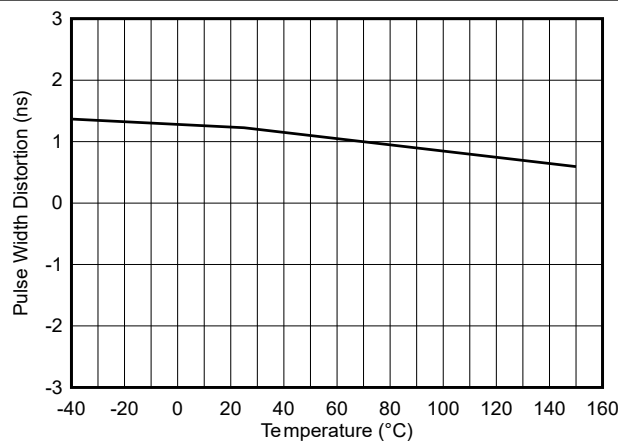
图 5-14. 脉宽失真度与温度之间的关系
