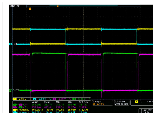
图 8-5. INA/B 和 OUTA/B 的台架测试波形
