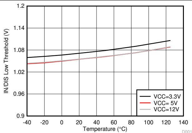
图 5-22. IN/DIS 低阈值
