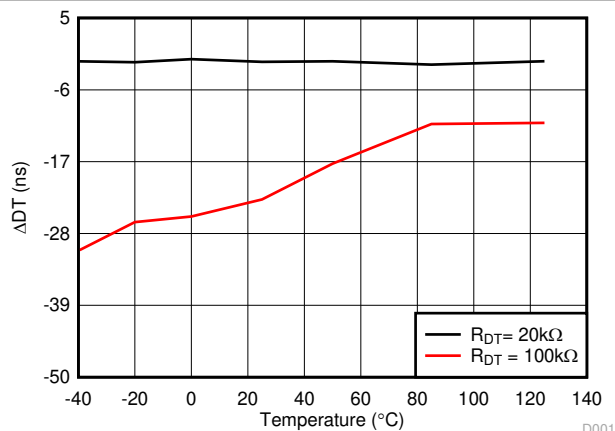
图 6-25. 死区时间匹配与温度之间的关系 ( R_{DT} = 20k\Omega 和 100k\Omega )
