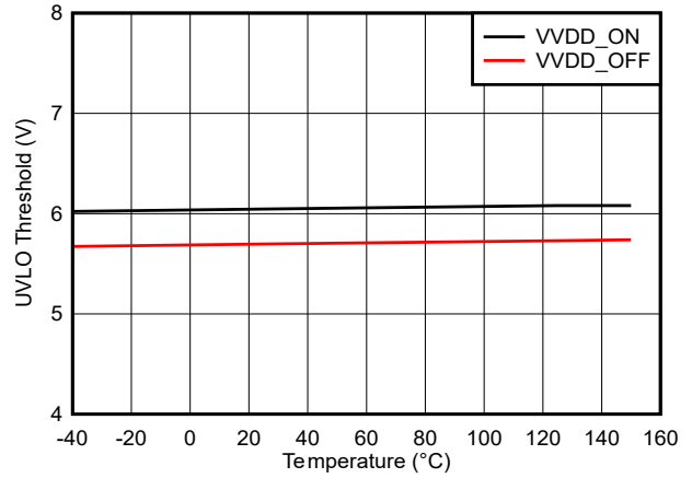
图 5-17. VDD 5V UVLO 阈值与温度间的关系
