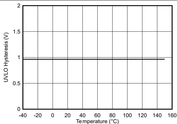
图 5-22. VDD 12V UVLO 迟滞与温度之间的关系
