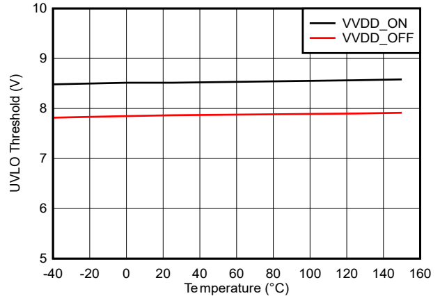
图 5-19. VDD 8V UVLO 阈值与温度间的关系
