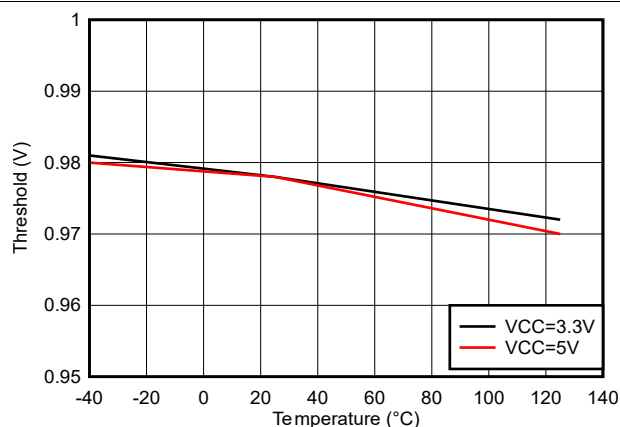
图 5-24. IN/DIS 低阈值
