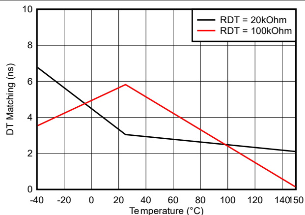
图 5-27. 死区时间匹配与温度之间的关系 ( R_{DT} = 20\text{k}\Omega 和 100\text{k}\Omega )
