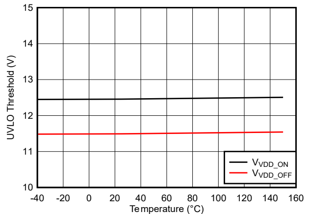
图 5-21. VDD 12V UVLO 阈值与温度间的关系
