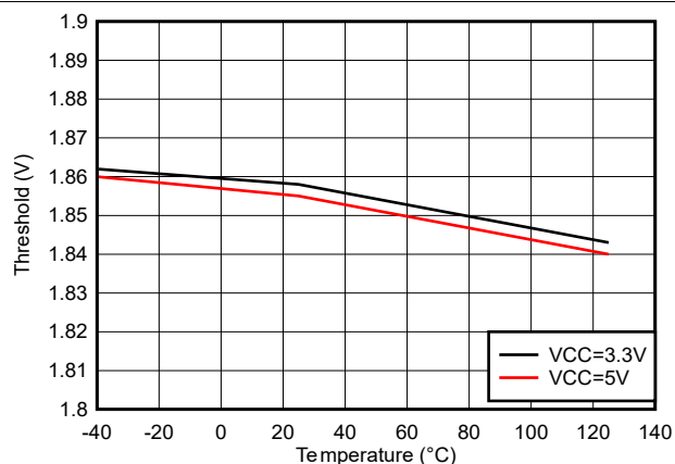
图 5-25. IN/DIS 高阈值
