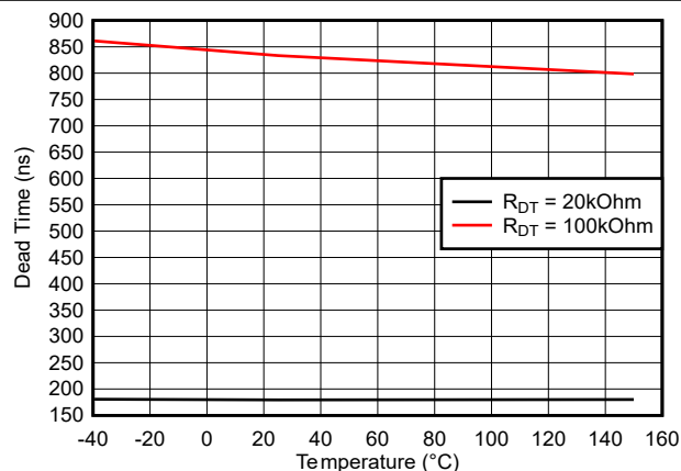
图 5-26. 死区时间与温度之间的关系 ( R_{DT} = 20\text{k}\Omega 和 100\text{k}\Omega )
