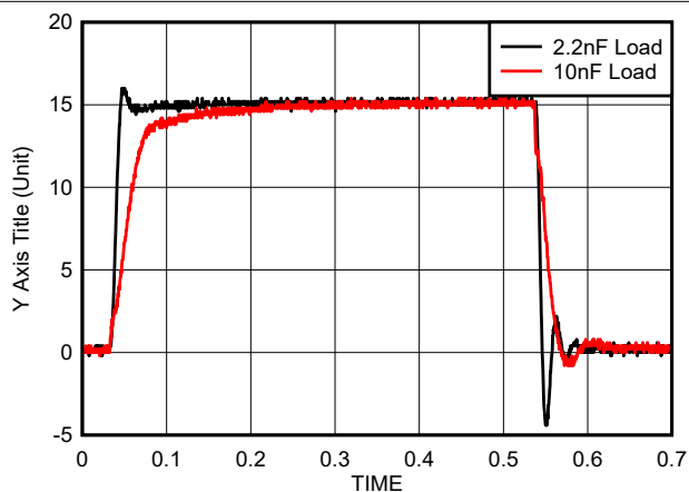
图 5-28. 典型输出波形
