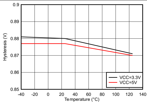
图 5-23. IN/DIS 迟滞与温度之间的关系
