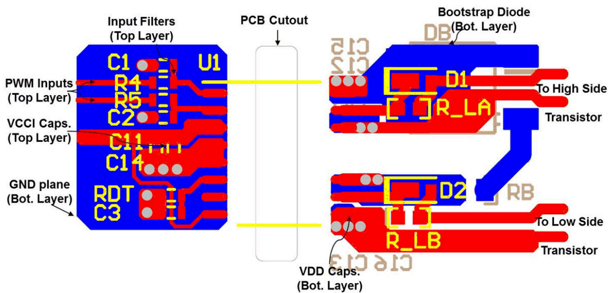
图 10-1. 布局示例
