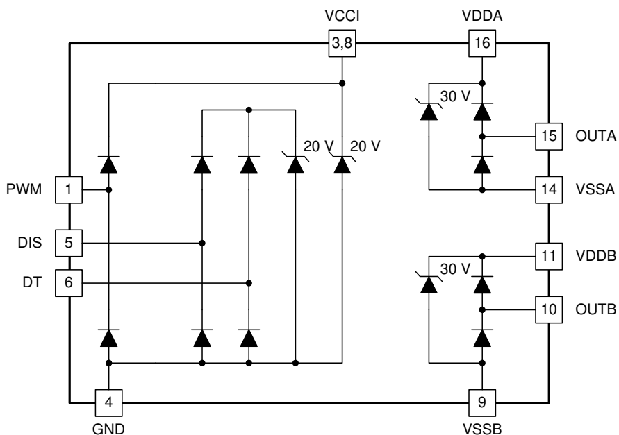
图 8-3. ESD Structure
