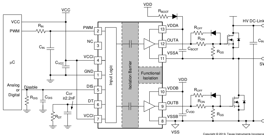
功能方框图
