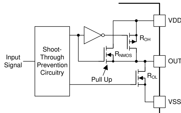
图 34. Output Stage
