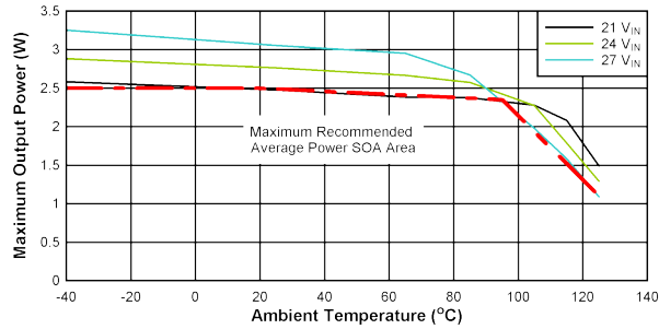
图 10-1. SOA 降额曲线：V VDD-VEE = 15V，V COM-VEE = 5V， T_{shut}=160^{\circ}\text{C} ，V COM-VEE 无负载。
