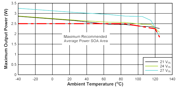
图 10-4. SOA 降额曲线：V VDD-VEE = 25V，V COM-VEE = 5V， T_{shut}=160^{\circ}\text{C} ，V COM-VEE 无负载。
