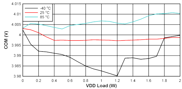
图 10-13. V_{COM-VEE} 负载调节: V_{IN} = 21V , V_{DD-VEE} = 22V , V_{COM-VEE} = 4V
