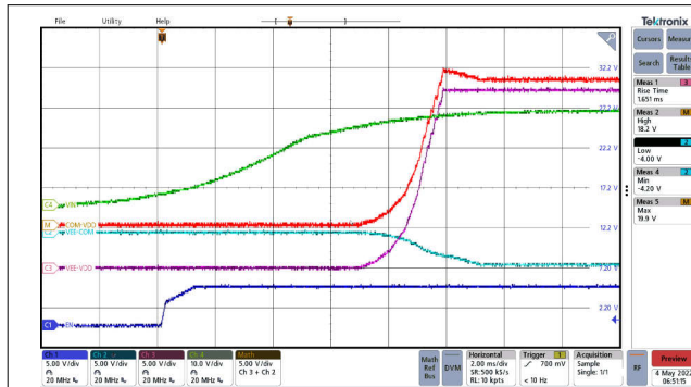
图 12-11. 上电序列。
