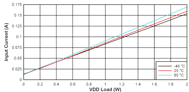
图 10-19. V_{DD-VEE} 上输入电流与负载间的关系: V_{IN} = 21V , V_{DD-VEE} = 22V , V_{COM-VEE} = 4V , V_{COM-VEE} 无负载
