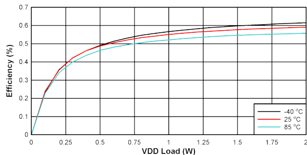
图 10-16. V_{DD-VEE} 上效率与负载间的关系: V_{IN} = 21V , V_{DD-VEE} = 22V , V_{COM-VEE} = 4V , V_{COM-VEE} 无负载
