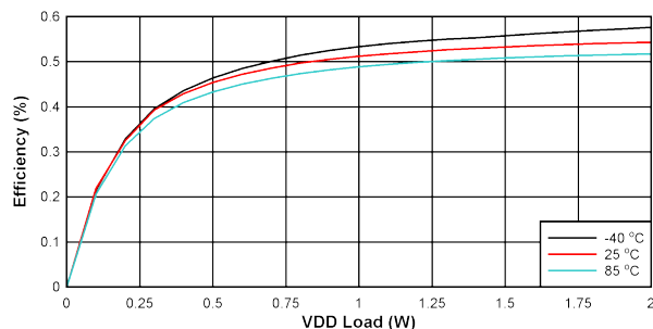
图 10-18. V_{DD-VEE} 上效率与负载间的关系: V_{IN} = 27V , V_{DD-VEE} = 22V , V_{COM-VEE} = 4V , V_{COM-VEE} 无负载
