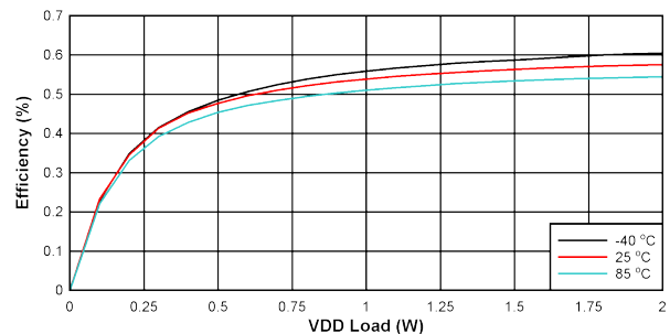
图 10-17. V_{DD-VEE} 上效率与负载间的关系: V_{IN} = 24V , V_{DD-VEE} = 22V , V_{COM-VEE} = 4V , V_{COM-VEE} 无负载
