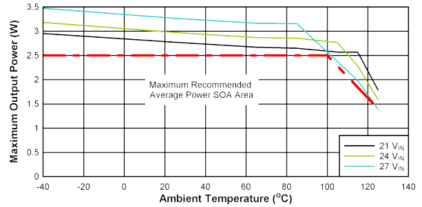
图 10-2. SOA 降额曲线：V VDD-VEE = 18V，V COM-VEE = 5V， T_{shut}=160^{\circ}\text{C} ，V COM-VEE 无负载。
