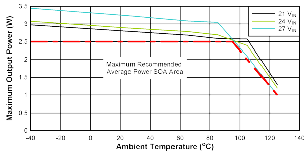
图 10-5. SOA 降额曲线：V VDD-VEE = 22V，V COM-VEE = 4V， T_{shut}=150^{\circ}\text{C} ，V COM-VEE 无负载，在屏蔽盒中测试。
