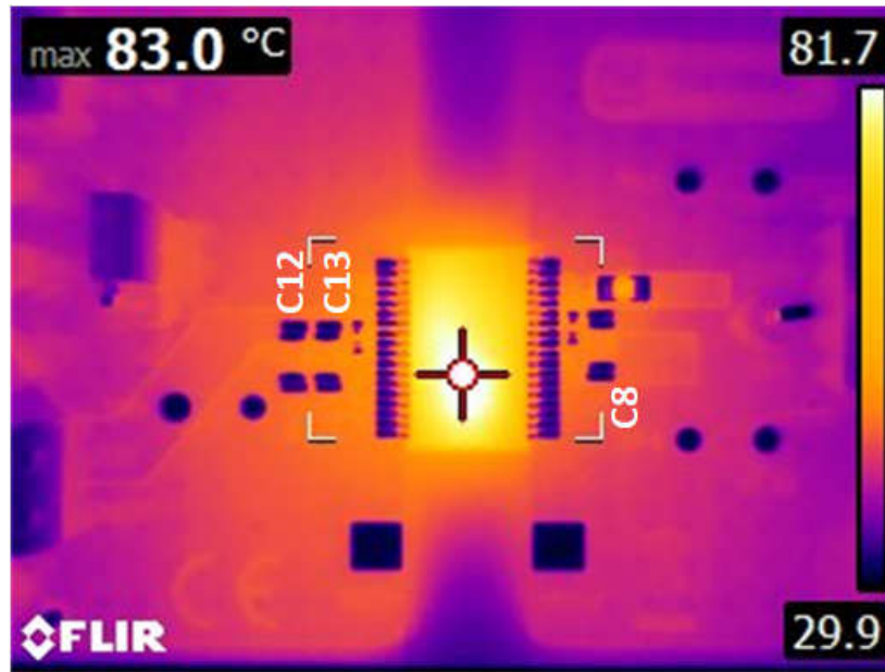
图 12-25. 热像图
