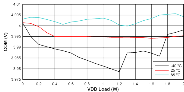
图 10-14. V_{COM-VEE} 负载调节: V_{IN} = 24V , V_{DD-VEE} = 22V , V_{COM-VEE} = 4V
