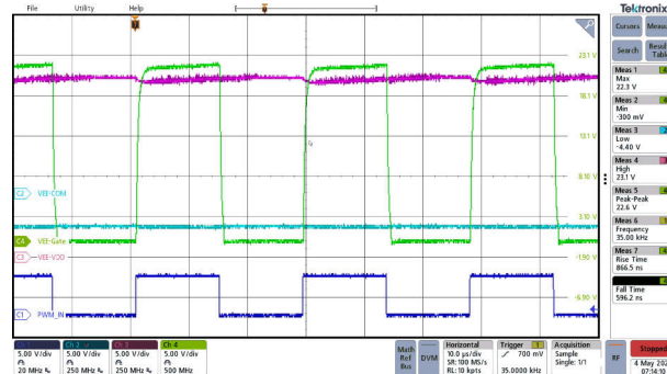
图 12-17. 在 35kHz 条件下开关 100nF 的栅极波形。
