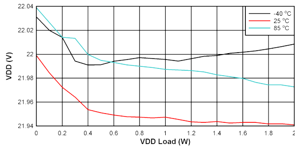
图 10-12. V_{DD-VEE} 负载调节: V_{IN} = 27V , V_{DD-VEE} = 22V , V_{COM-VEE} = 4V
