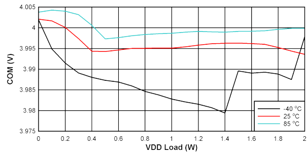
图 10-15. V_{COM-VEE} 负载调节: V_{IN} = 27V , V_{DD-VEE} = 22V , V_{COM-VEE} = 4V
