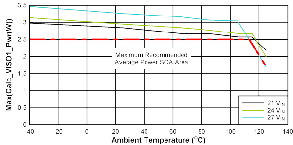
图 10-3. SOA 降额曲线：V VDD-VEE = 22V，V COM-VEE = 4V， T_{shut}=160^{\circ}\text{C} ，V COM-VEE 无负载。
