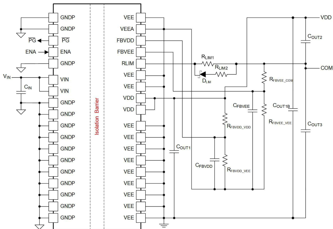
图 12-8. 配置为 V_{COM\_VEE} 调节 > 2.5V 时的双路输出应用原理图
