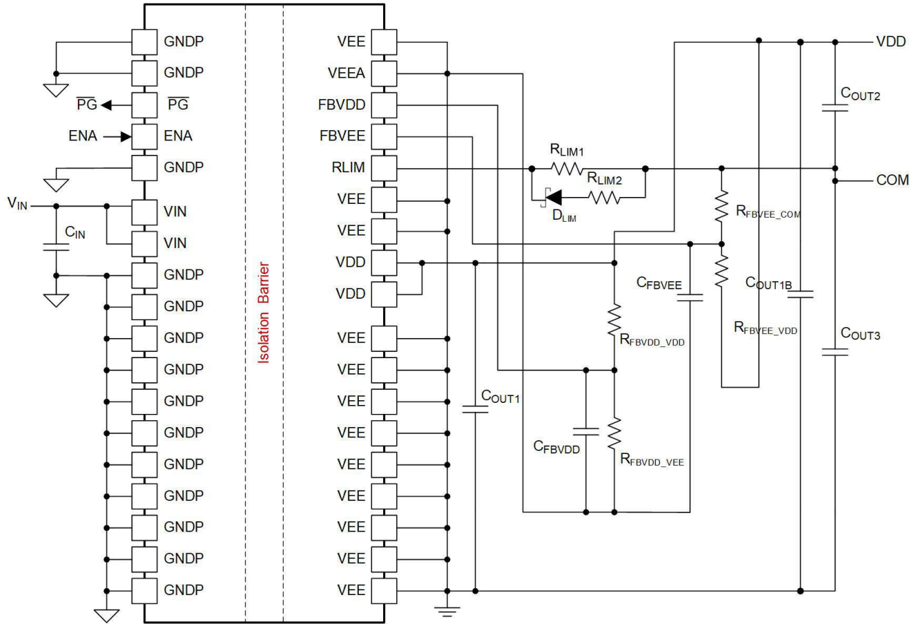
图 12-10. 配置为 V_{\text{COM\_VEE}} 调节 < 2.5\text{V} 时的双路输出应用原理图
