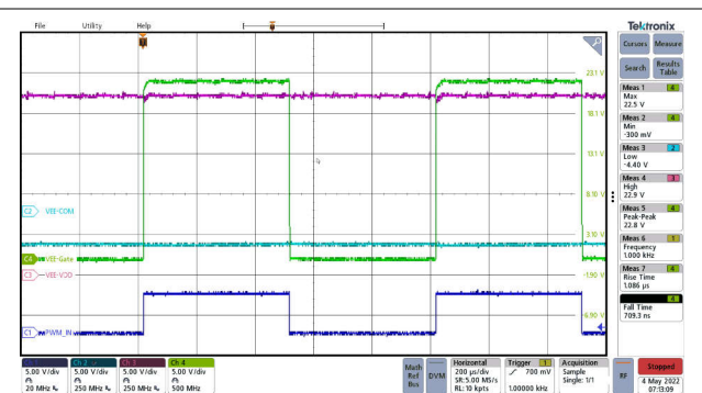
图 12-16. 在 1kHz 条件下开关 100nF 的栅极波形。
