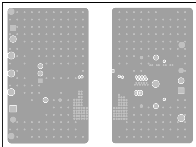
图 8-23. UCC14341-Q1EVM，信号层 3 (与第 2 层相同)
