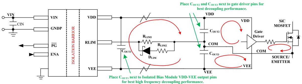
图 8-3. 具有 C_{out1} 、 C_{out2} 和 C_{out3} 的双路输出原理图
