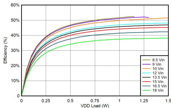
图 6-30. UCC14341B-Q1 V_{VDD-VEE} 上效率与负载间的关系: T_{AMBIENT} = -40^{\circ}C , V_{VDD-VEE} = 15V , V_{COM-VEE} = 4V , V_{COM-VEE} 无负载
