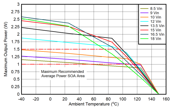
图 6-26. UCC14341B-Q1 SOA 降额曲线: V_{VDD-VEE} = 15V , V_{COM-VEE} = 5V , T_{shut} = 160^{\circ}C , V_{COM-VEE} 无负载
