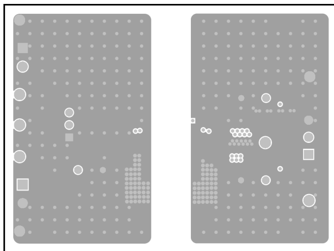
图 8-22. UCC14341-Q1EVM , 信号层 2 ( 与第 3 层相同 )
