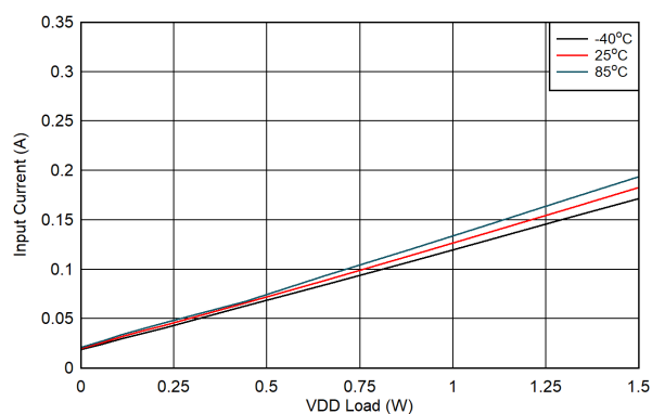
图 6-25. V_{DD-VEE} 上输入电流与负载间的关系: V_{IN} = 18V , V_{DD-VEE} = 22V , V_{COM-VEE} = 4V , V_{COM-VEE} 无负载
