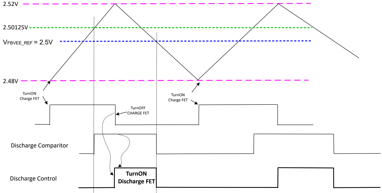
图 7-3. COM-VEE 电压调节图
