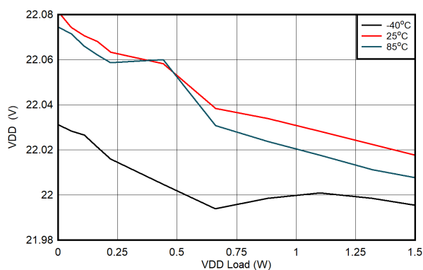
图 6-13. V_{VDD-VEE} 负载调节: V_{IN} = 18V , V_{VDD-VEE} = 22V , V_{COM-VEE} = 4V
