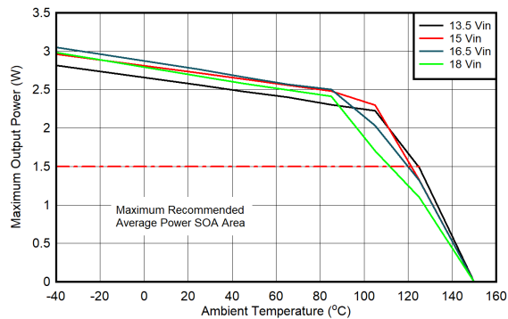
图 6-4. SOA 降额曲线: V_{DD-VEE} = 22\text{V} , V_{COM-VEE} = 4\text{V} , T_{shut} = 160^{\circ}\text{C} , V_{COM-VEE} 无负载
