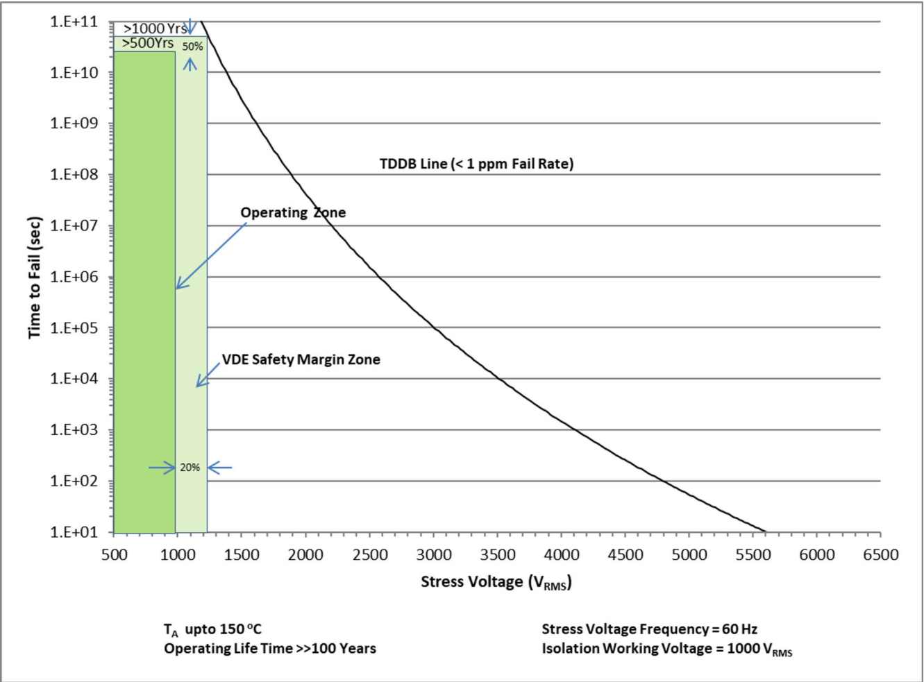
图 6-1. TDDB : 1000Vrms 工作电压下的绝缘寿命预测。
