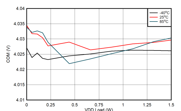
图 6-17. V_{COM-VEE} 负载调节: V_{IN} = 18V , V_{DD-VEE} = 22V , V_{COM-VEE} = 4V
