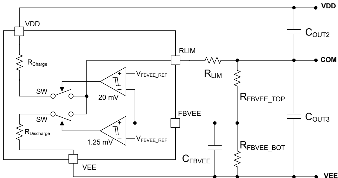
图 7-2. COM-VEE 电压调节
