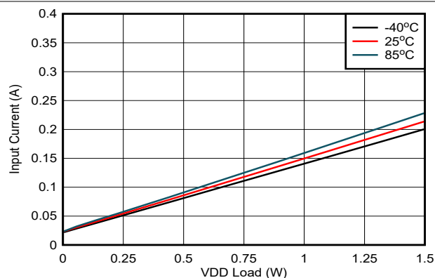
图 6-22. V_{DD-VEE} 上输入电流与负载间的关系: V_{IN} = 13.5V , V_{DD-VEE} = 22V , V_{COM-VEE} = 4V , V_{COM-VEE} 无负载
