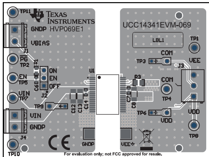
图 8-21. UCC14341-Q1EVM , PCB 顶层, 组装
