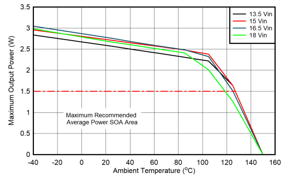
图 6-5. SOA 降额曲线: V_{DD-VEE} = 25\text{V} , V_{COM-VEE} = 5\text{V} , T_{shut} = 160^{\circ}\text{C} , V_{COM-VEE} 无负载
