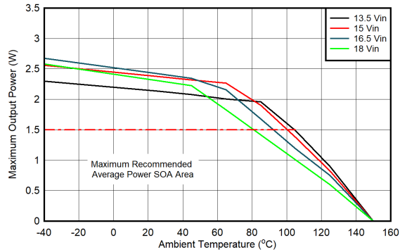
图 6-2. SOA 降额曲线: V_{DD-VEE} = 15\text{V} , V_{COM-VEE} = 5\text{V} , T_{shut} = 160^{\circ}\text{C} , V_{COM-VEE} 无负载
