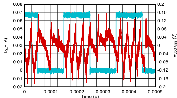
图 6-9. 负载瞬态响应: 在空载和 1.5W 之间, V_{IN} = 15V , V_{VDD-VEE} = 22V , V_{COM-VEE} = 4V
