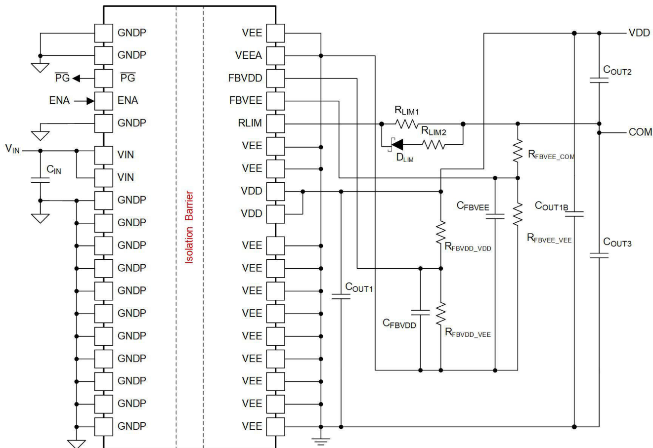
图 8-8. 配置为 V_{COM\_VEE} 调节 > 2.5V 时的双路输出应用原理图
