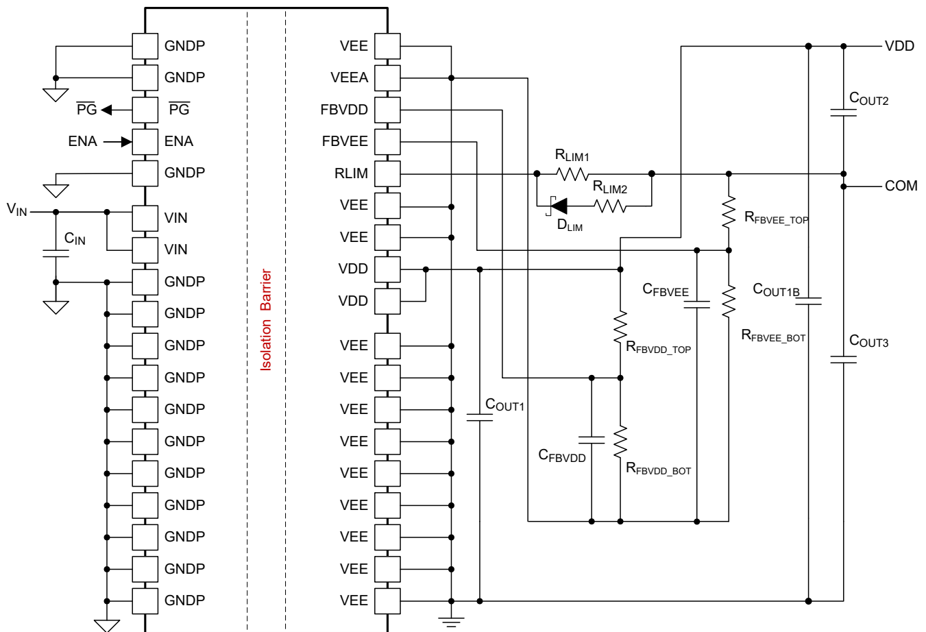
图 8-1. 双路可调输出配置
