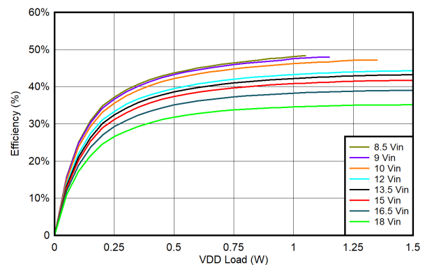
图 6-31. UCC14341B-Q1 V_{VDD-VEE} 上效率与负载间的关系: T_{AMBIENT} = 25^{\circ}C , V_{VDD-VEE} = 15V , V_{COM-VEE} = 4V , V_{COM-VEE} 无负载
