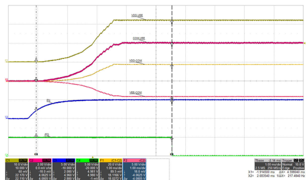
图 6-7. 启动: V_{IN} = 15\text{V} , V_{DD-VEE} = 22\text{V} , V_{COM-VEE} = 4\text{V} , I_{VDD-VEE} = 68\text{mA} , V_{COM-VEE} 无负载。时间标度: 1ms/div。
