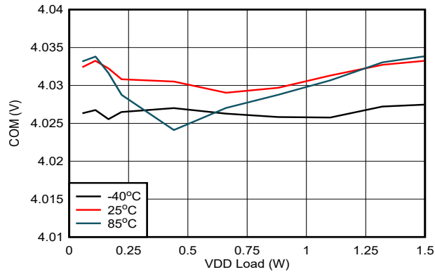
图 6-16. V_{COM-VEE} 负载调节: V_{IN} = 16.5V , V_{DD-VEE} = 22V , V_{COM-VEE} = 4V
