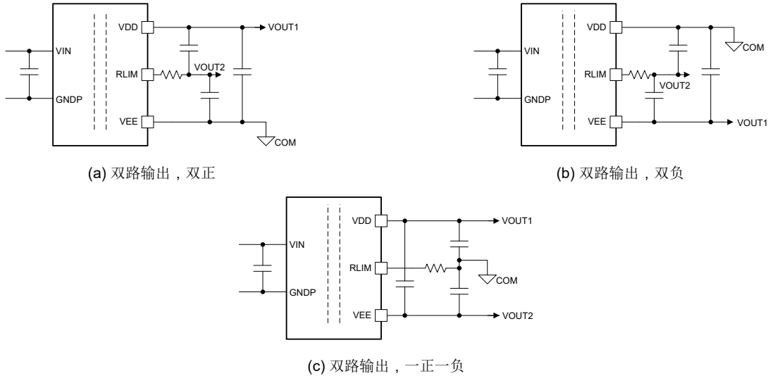
图 8-6. 双路输出配置
