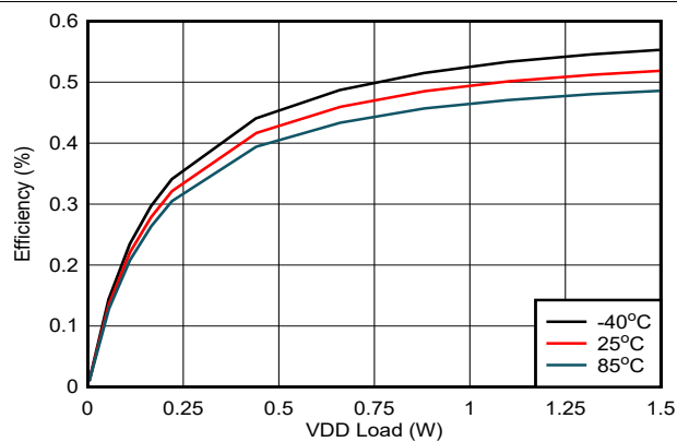
图 6-18. V_{DD-VEE} 上效率与负载间的关系: V_{IN} = 13.5V , V_{DD-VEE} = 22V , V_{COM-VEE} = 4V , V_{COM-VEE} 无负载
