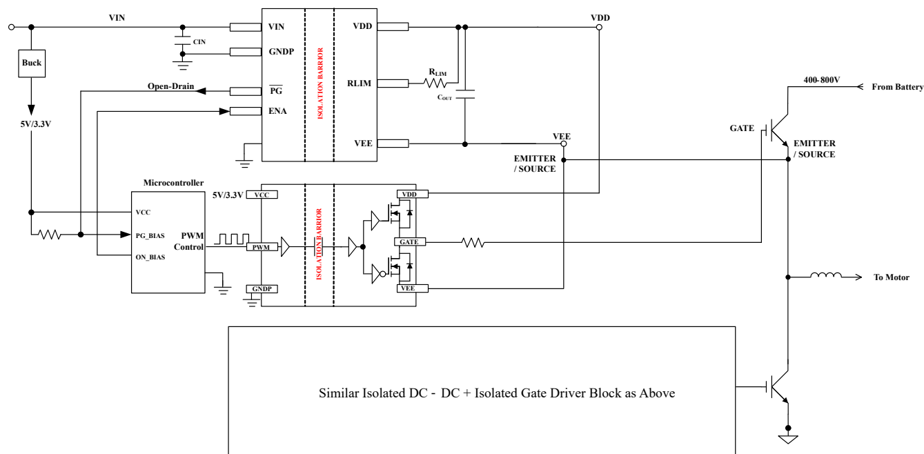
图 8-12. 单输出系统配置
