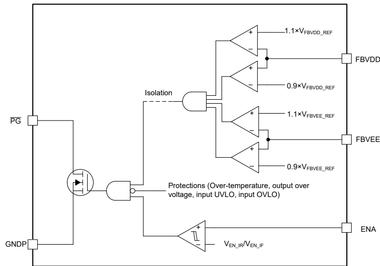
图 7-7. \overline{\text{PG}} 引脚逻辑
