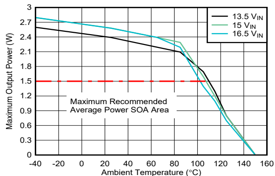
图 6-6. SOA 降额曲线: V_{DD-VEE} = 22\text{V} , V_{COM-VEE} = 4\text{V} , T_{shut} = 150^{\circ}\text{C} , V_{COM-VEE} 无负载, 在屏蔽盒中测试。
