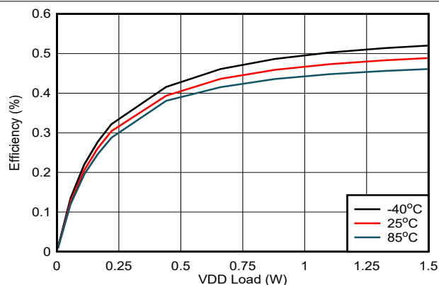
图 6-20. V_{DD-VEE} 上效率与负载间的关系: V_{IN} = 16.5V , V_{DD-VEE} = 22V , V_{COM-VEE} = 4V , V_{COM-VEE} 无负载
