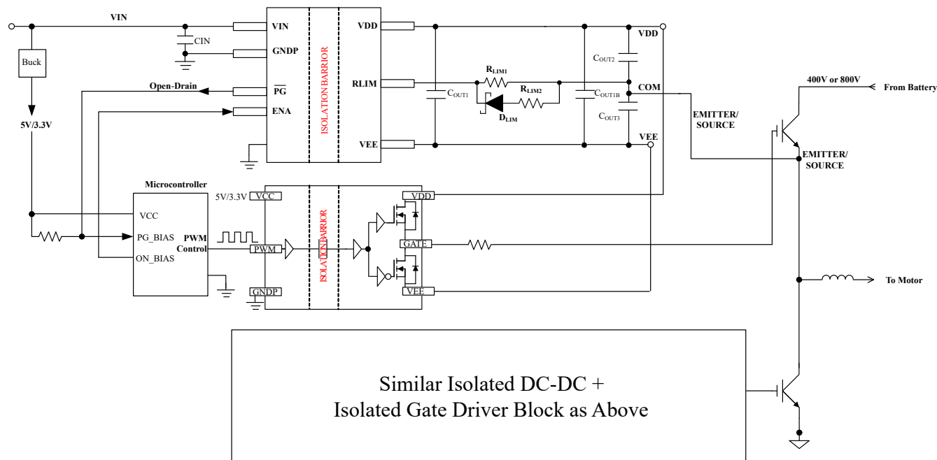
图 8-11. 双输出系统配置
