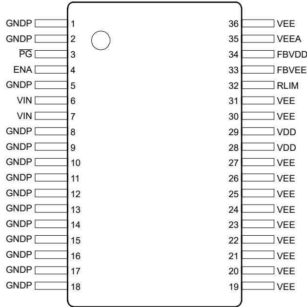
图 5-1. DWN 封装，36 引脚 SSOP (顶视图)
