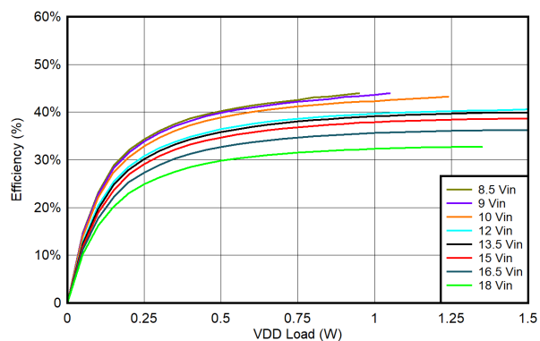
图 6-32. UCC14341B-Q1 V_{VDD-VEE} 上效率与负载间的关系: T_{AMBIENT} = 85^{\circ}\text{C} , V_{VDD-VEE} = 15\text{V} , V_{COM-VEE} = 4\text{V} , V_{COM-VEE} 无负载
