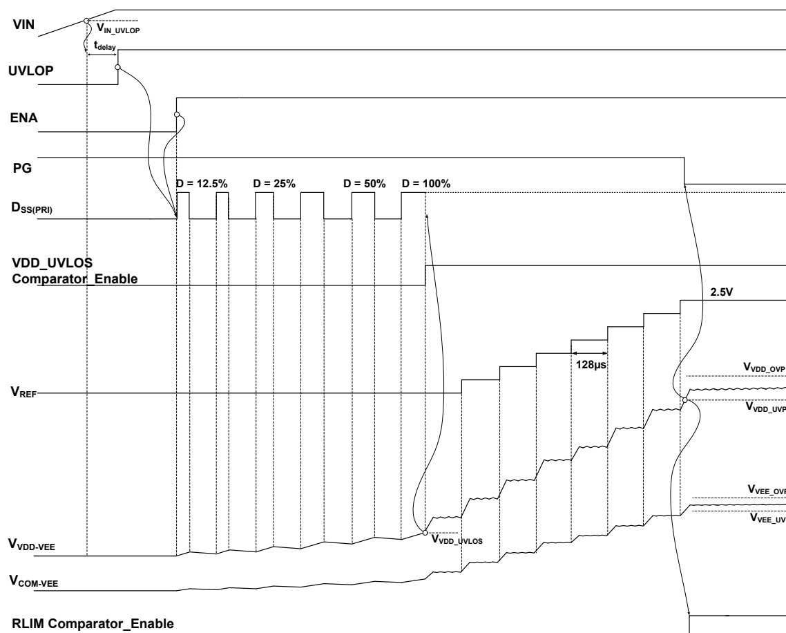
图 7-5. 输出电压软启动图
