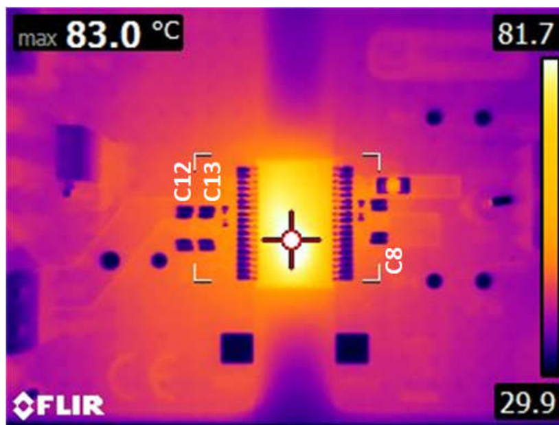
图 8-18. 热像图
