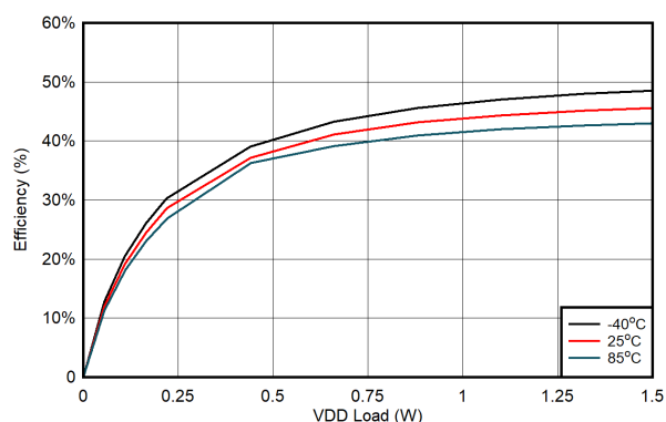
图 6-21. V_{DD-VEE} 上效率与负载间的关系: V_{IN} = 18V , V_{DD-VEE} = 22V , V_{COM-VEE} = 4V , V_{COM-VEE} 无负载
