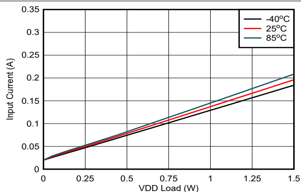
图 6-23. V_{DD-VEE} 上输入电流与负载间的关系: V_{IN} = 15V , V_{DD-VEE} = 22V , V_{COM-VEE} = 4V , V_{COM-VEE} 无负载
