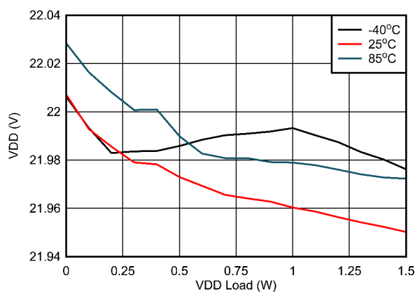
图 6-10. V_{VDD-VEE} 负载调节: V_{IN} = 13.5V , V_{VDD-VEE} = 22V , V_{COM-VEE} = 4V
