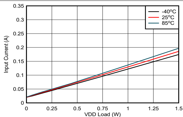
图 6-24. V_{DD-VEE} 上输入电流与负载间的关系: V_{IN} = 16.5V , V_{DD-VEE} = 22V , V_{COM-VEE} = 4V , V_{COM-VEE} 无负载
