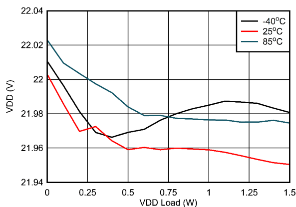
图 6-12. V_{VDD-VEE} 负载调节: V_{IN} = 16.5V , V_{VDD-VEE} = 22V , V_{COM-VEE} = 4V
