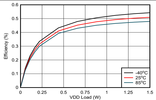
图 6-19. V_{DD-VEE} 上效率与负载间的关系: V_{IN} = 15V , V_{DD-VEE} = 22V , V_{COM-VEE} = 4V , V_{COM-VEE} 无负载
