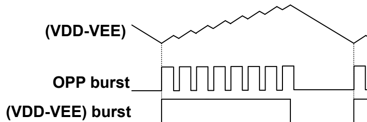
图 7-4. 带小型突发的过功率保护示意图
