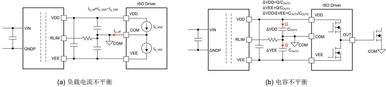
图 8-7. 电压不平衡来源
