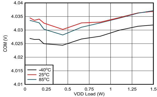
图 6-14. V_{COM-VEE} 负载调节: V_{IN} = 13.5V , V_{DD-VEE} = 22V , V_{COM-VEE} = 4V
