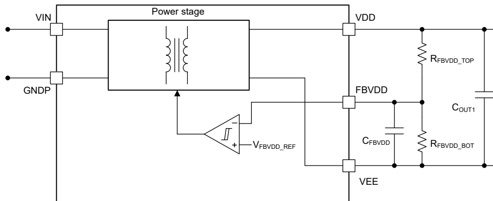
图 7-1. VDD-VEE 电压调节
