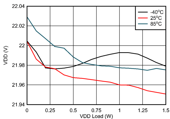
图 6-11. V_{VDD-VEE} 负载调节: V_{IN} = 15V , V_{VDD-VEE} = 22V , V_{COM-VEE} = 4V
