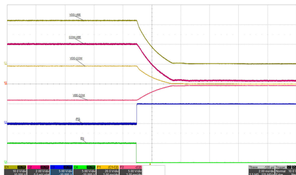
图 6-8. 关断: V_{IN} = 15V , V_{VDD-VEE} = 22V , V_{COM-VEE} = 4V , I_{VDD-VEE} = 68mA , V_{COM-VEE} 无负载。时间标度: 2ms/div。
