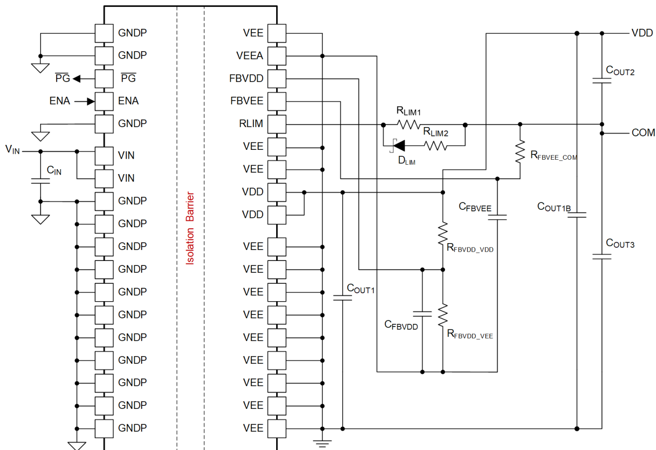
图 8-9. 配置为 V_{COM\_VEE} 调节 = 2.5V 时的双路输出应用原理图
