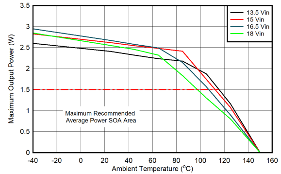
图 6-3. SOA 降额曲线: V_{DD-VEE} = 18\text{V} , V_{COM-VEE} = 3\text{V} , T_{shut} = 160^{\circ}\text{C} , V_{COM-VEE} 无负载
