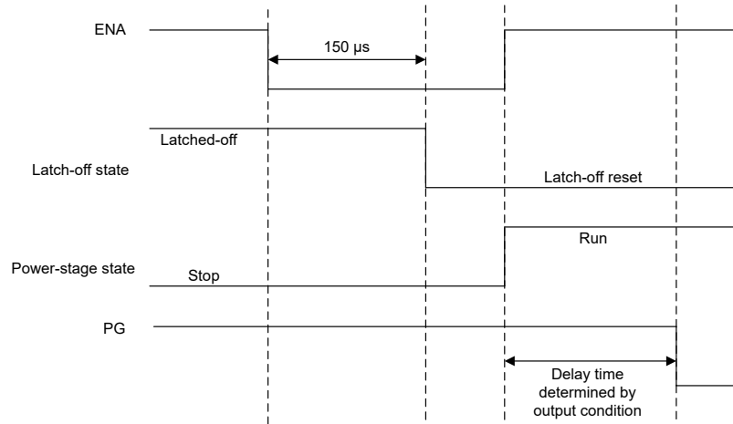
图 7-6. 使用 ENA 引脚的闭锁复位
