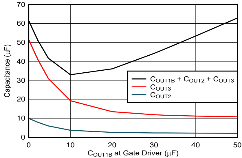
图 8-5. 输出电容随 C_{OUT1B} 选择的变化
