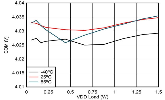
图 6-15. V_{COM-VEE} 负载调节: V_{IN} = 15V , V_{DD-VEE} = 22V , V_{COM-VEE} = 4V
