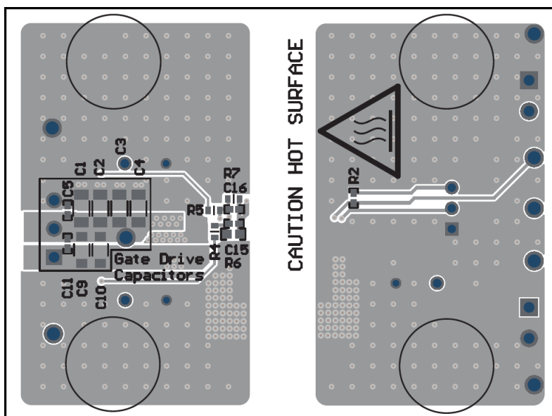
图 8-24. UCC14341-Q1EVM，PCB 底层，组装 (镜像视图)
