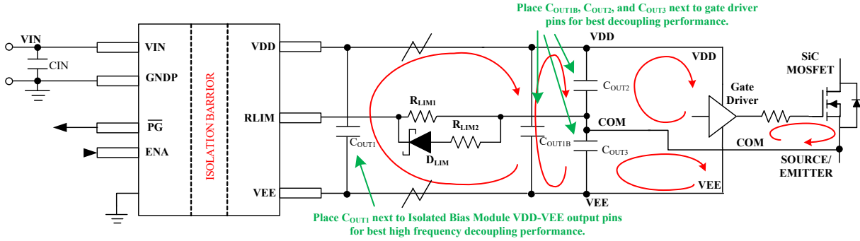
图 8-4. 具有 C_{OUT1} 、 C_{OUT1B} 、 C_{OUT2} 和 C_{OUT3} 的双路输出原理图
