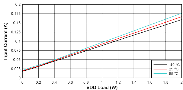
图 10-19. V_{D\overline{D}-VEE} 上输入电流与负载间的关系: V_{IN} = 21V , V_{D\overline{D}-VEE} = 22V , V_{COM-VEE} = 4V , V_{COM-VEE} 无负载
