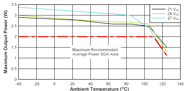
图 10-3. SOA 降额曲线： V_{DD-VEE} = 22\text{V} ， V_{COM-VEE} = 4\text{V} ， T_{shut}=150^{\circ}\text{C} ， V_{COM-VEE} 无负载。
