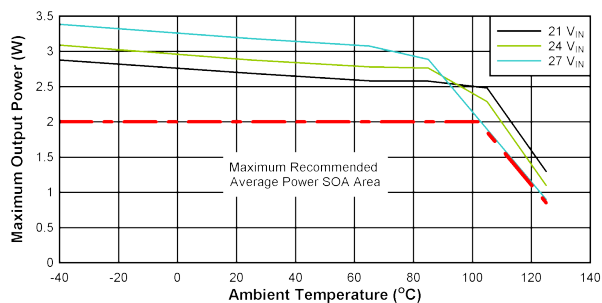
图 10-2. SOA 降额曲线： V_{DD-VEE} = 18\text{V} ， V_{COM-VEE} = 5\text{V} ， T_{shut}=150^{\circ}\text{C} ， V_{COM-VEE} 无负载。
