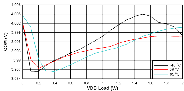
图 10-13. V_{COM-VEE} 负载调节: V_{IN} = 21V , V_{D\overline{D}-VEE} = 22V , V_{COM-VEE} = 4V
