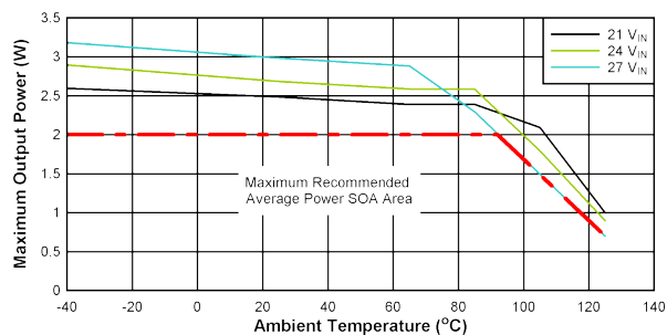
图 10-1. SOA 降额曲线： V_{DD-VEE} = 15\text{V} ， V_{COM-VEE} = 5\text{V} ， T_{shut}=150^{\circ}\text{C} ， V_{COM-VEE} 无负载。
