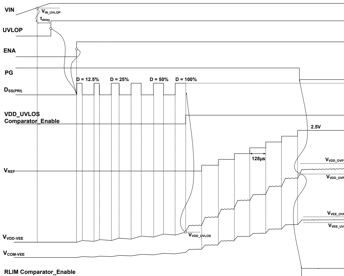
图 11-5. 输出电压软启动图
