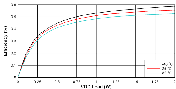
图 10-17. V_{D\overline{D}-VEE} 上效率与负载间的关系: V_{IN} = 24V , V_{D\overline{D}-VEE} = 22V , V_{COM-VEE} = 4V , V_{COM-VEE} 无负载
