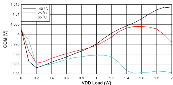
图 10-15. V_{COM-VEE} 负载调节: V_{IN} = 27V , V_{D\overline{D}-VEE} = 22V , V_{COM-VEE} = 4V
