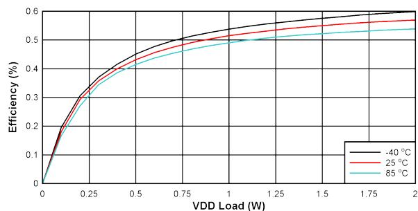
图 10-16. V_{D\overline{D}-VEE} 上效率与负载间的关系: V_{IN} = 21V , V_{D\overline{D}-VEE} = 22V , V_{COM-VEE} = 4V , V_{COM-VEE} 无负载
