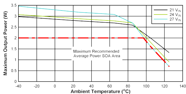
图 10-5. SOA 降额曲线： V_{DD-VEE} = 22\text{V} ， V_{COM-VEE} = 4\text{V} ， T_{shut}=140^{\circ}\text{C} ， V_{COM-VEE} 无负载，在屏蔽盒中测试。
