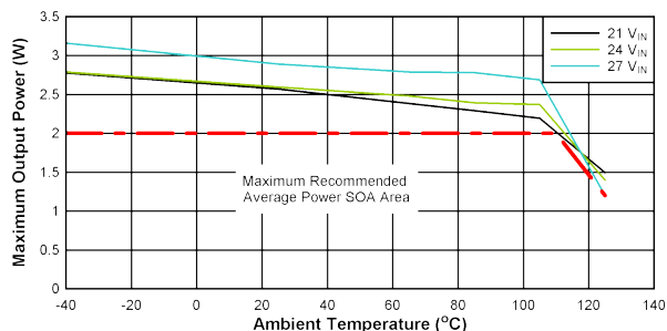
图 10-4. SOA 降额曲线： V_{DD-VEE} = 25\text{V} ， V_{COM-VEE} = 5\text{V} ， T_{shut}=150^{\circ}\text{C} ， V_{COM-VEE} 无负载。
