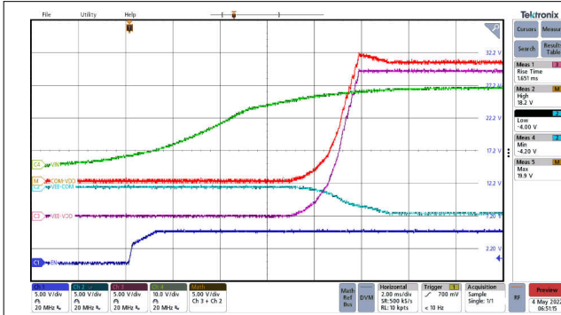
图 12-11. 上电序列。
