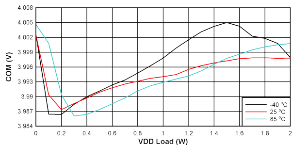
图 10-14. V_{COM-VEE} 负载调节: V_{IN} = 24V , V_{D\overline{D}-VEE} = 22V , V_{COM-VEE} = 4V
