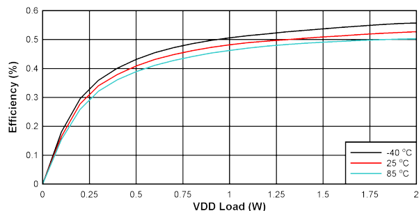
图 10-18. V_{D\overline{D}-VEE} 上效率与负载间的关系: V_{IN} = 27V , V_{D\overline{D}-VEE} = 22V , V_{COM-VEE} = 4V , V_{COM-VEE} 无负载
