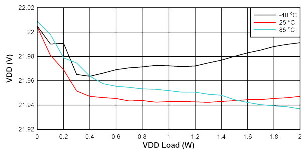
图 10-12. V_{D\overline{D}-VEE} 负载调节: V_{IN} = 27V , V_{D\overline{D}-VEE} = 22V , V_{COM-VEE} = 4V
