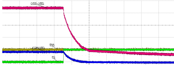
图 7-8. 关断: V_{IN} = 12V , V_{VDD-VEE} = 22V , V_{COM-VEE} = 4V , V_{COM-VEE} 无负载。电压标度: 5V/div, 时间标度: 50ms/div。
