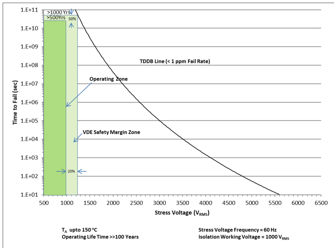
图 9-1. TDDDB : 1000Vrms 工作电压下的绝缘寿命预测。
