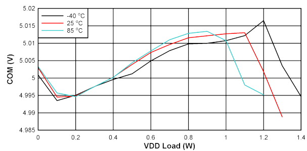
图 10-11. V_{COM-VEE} 负载调节: V_{IN} = 10V , V_{DD-VEE} = 12V , V_{COM-VEE} = 5V
