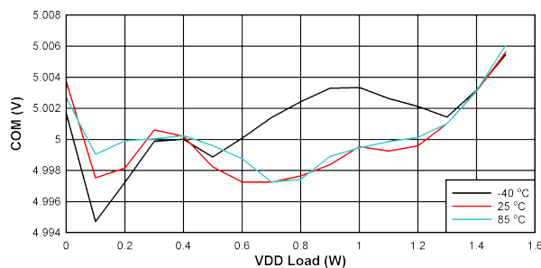
图 10-12. V_{COM-VEE} 负载调节: V_{IN} = 12V , V_{DD-VEE} = 12V , V_{COM-VEE} = 5V
