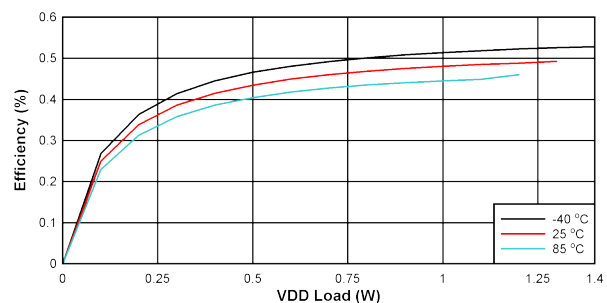
图 10-15. V_{DD-VEE} 上效率与负载间的关系: V_{IN} = 10V , V_{DD-VEE} = 12V , V_{COM-VEE} = 5V , V_{COM-VEE} 无负载
