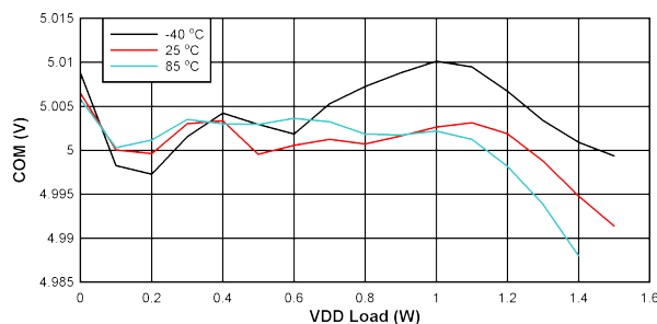
图 10-14. V_{COM-VEE} 负载调节: V_{IN} = 18V , V_{DD-VEE} = 12V , V_{COM-VEE} = 5V
