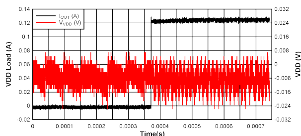
图 10-6. 负载瞬态响应：无负载至 1W, V_{IN} = 12V , V_{DD-VEE} = 12V , V_{COM-VEE} = 5V
