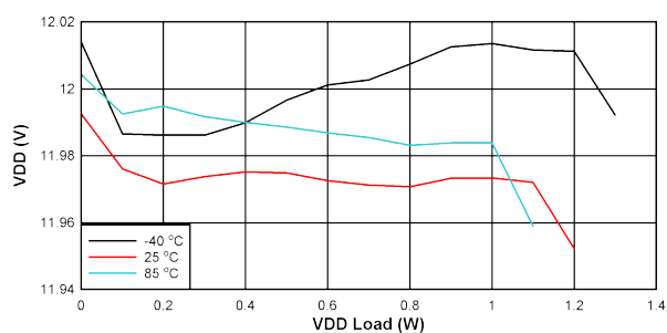
图 10-7. V_{DD-VEE} 负载调节： V_{IN} = 10V , V_{DD-VEE} = 12V , V_{COM-VEE} = 5V
