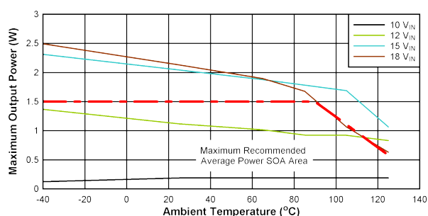
图 10-4. SOA 降额曲线： V_{DD-VEE} = 18V , V_{COM-VEE} = 5V , T_{shut}=160^{\circ}C , V_{COM-VEE} 无负载。
