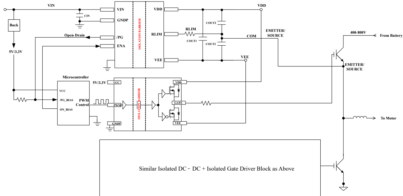
图 12-11. 双输出系统配置
