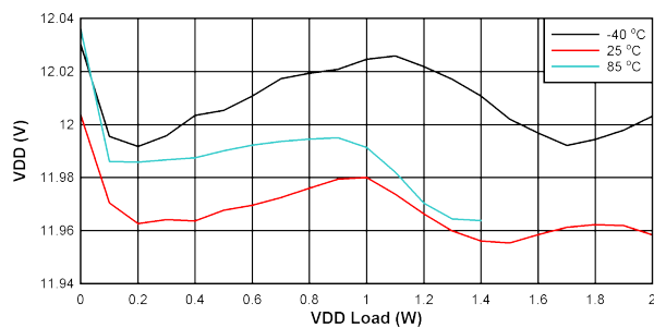
图 10-10. V_{DD-VEE} 负载调节: V_{IN} = 18V , V_{DD-VEE} = 12V , V_{COM-VEE} = 5V
