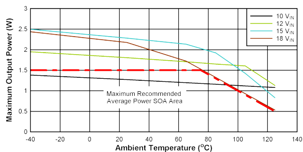
图 10-2. SOA 降额曲线： V_{DD-VEE} = 12V , V_{COM-VEE} = 5V , T_{shut}=160^{\circ}C , V_{COM-VEE} 无负载。
