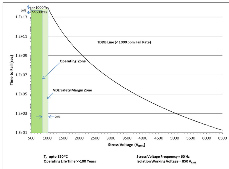
图 9-1. TDDDB：850Vrms 工作电压下的绝缘寿命预测。
