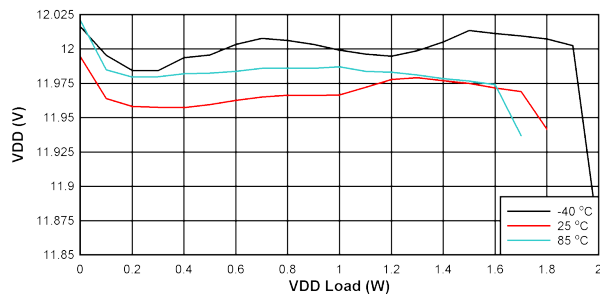
图 10-8. V_{DD-VEE} 负载调节: V_{IN} = 12V , V_{DD-VEE} = 12V , V_{COM-VEE} = 5V
