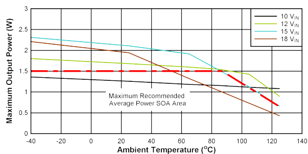
图 10-1. SOA 降额曲线： V_{DD-VEE} = 10V , V_{COM-VEE} = 5V , T_{shut}=160^{\circ}C , V_{COM-VEE} 无负载。
