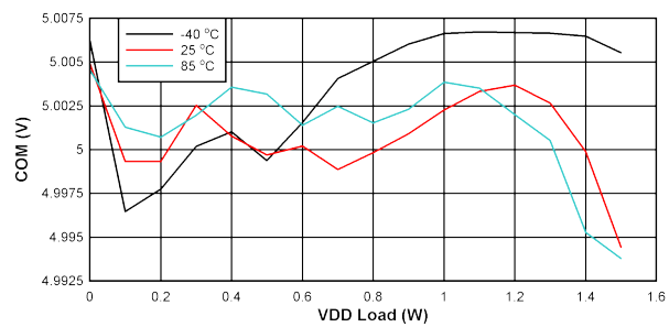
图 10-13. V_{COM-VEE} 负载调节: V_{IN} = 15V , V_{DD-VEE} = 12V , V_{COM-VEE} = 5V
