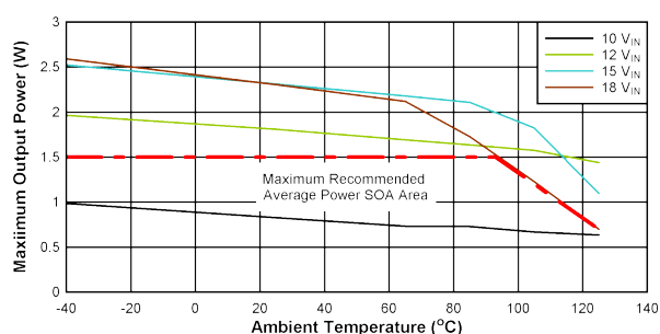
图 10-3. SOA 降额曲线： V_{DD-VEE} = 15V , V_{COM-VEE} = 5V , T_{shut}=160^{\circ}C , V_{COM-VEE} 无负载。
