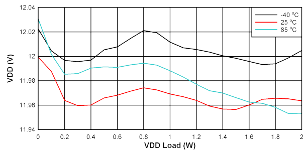
图 10-9. V_{DD-VEE} 负载调节: V_{IN} = 15V , V_{DD-VEE} = 12V , V_{COM-VEE} = 5V
