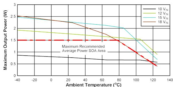
图 10-5. SOA 降额曲线： V_{DD-VEE} = 15V , V_{COM-VEE} = 5V , T_{shut}=150^{\circ}C , V_{COM-VEE} 无负载，在屏蔽盒中测试。
