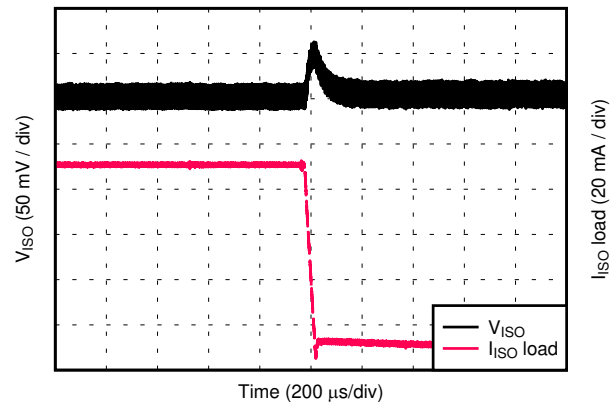
图 8-13. V_{ISO} Load Transient Response, 90% to 10% Load Step, 5.0-V Input, 5.0-V Output
