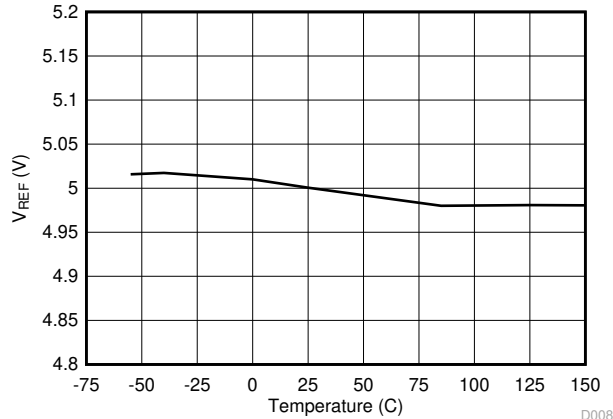
图 6-7. VREF 电压与温度间的关系
