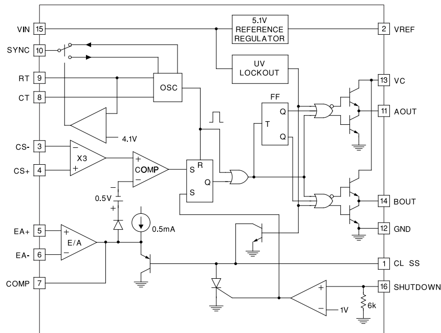
方框图
