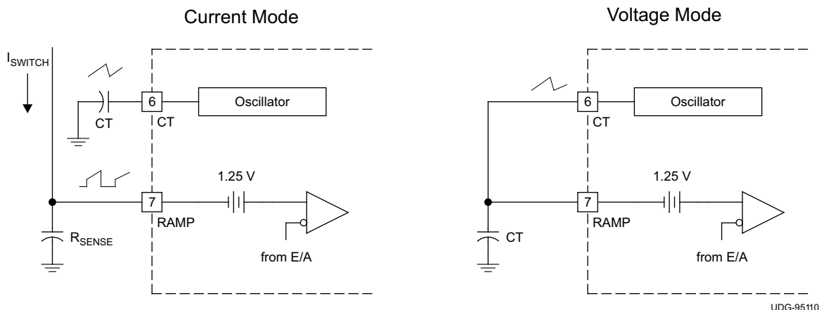
图 7-1. Control Methods
