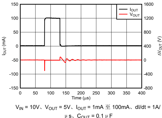
图 7-7. 负载瞬态特性 (M3 版本)
