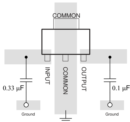
图 7-9. 布局图
