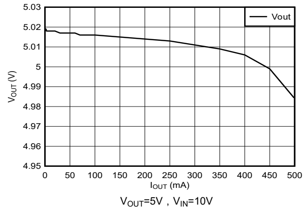
图 5-2. T_J = 25^\circ\text{C} 时的负载调整 (M3 版本)
