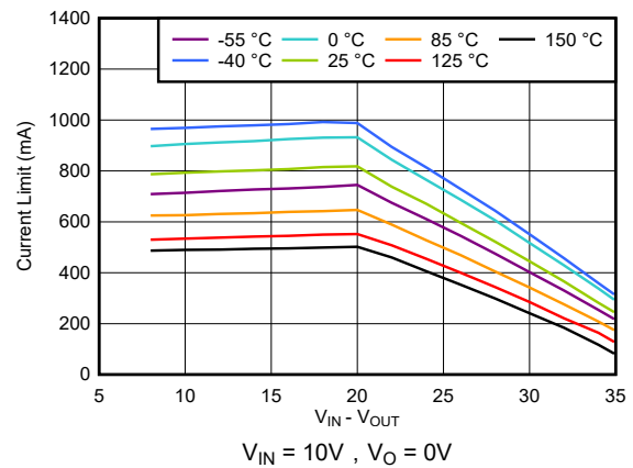
图 5-6. I_{CL} 与输入电压间的关系 (M3 版本)
