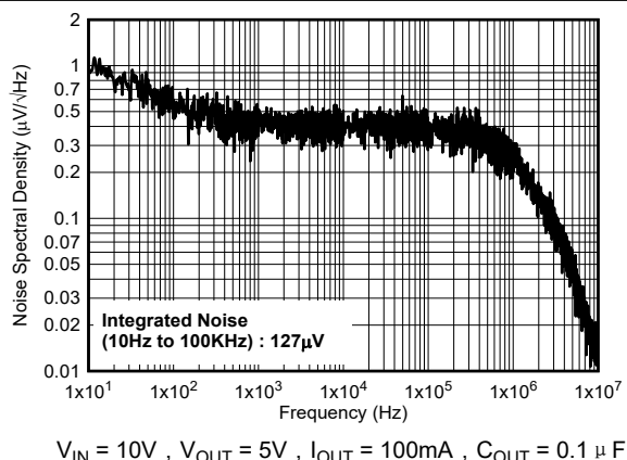
图 5-10. 噪声与频率间的关系 (M3 版本)
