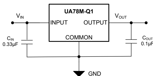
图 7-1. 固定输出稳压器
