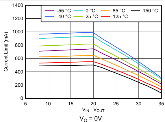
图 5-6. I_{CL} vs Input Voltage (New Chip)
