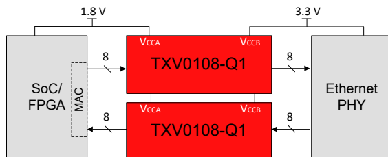
RGMII 应用中的 TXV0108-Q1
