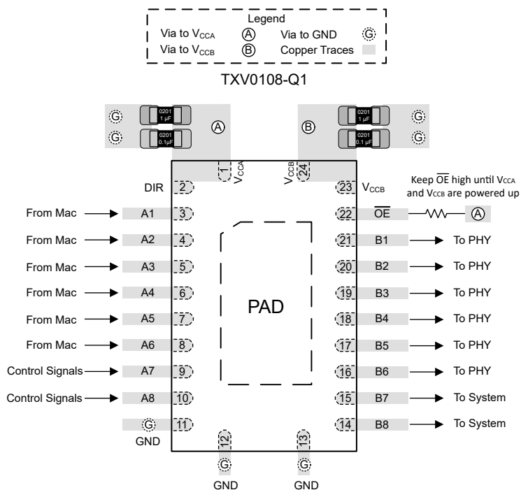
图 8-6. 布局示例 - TXV0108-Q1
