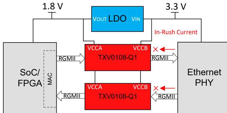
图 8-5. 使用 TXV0108-Q1 进行电源隔离
