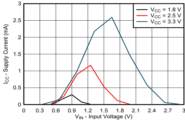
图 5-1. 电源电流与输入电压电源间的关系 (上升)
