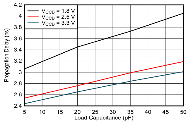
图 5-6. 传播延迟 T_{PLH} 与负载电容间的关系 ( V_{CCB} = 1.8\text{V} )
