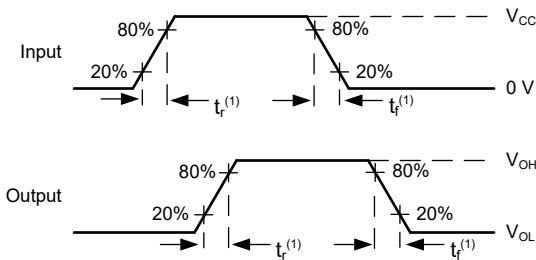
图 6-3. 输入转换上升或下降速率
