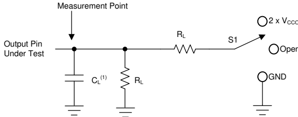
图 6-1. 负载电路
