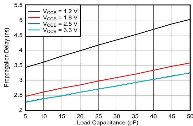
图 5-5. 传播延迟 T_{PLH} 与负载电容间的关系 ( V_{CCB} = 1.2\text{V} )
