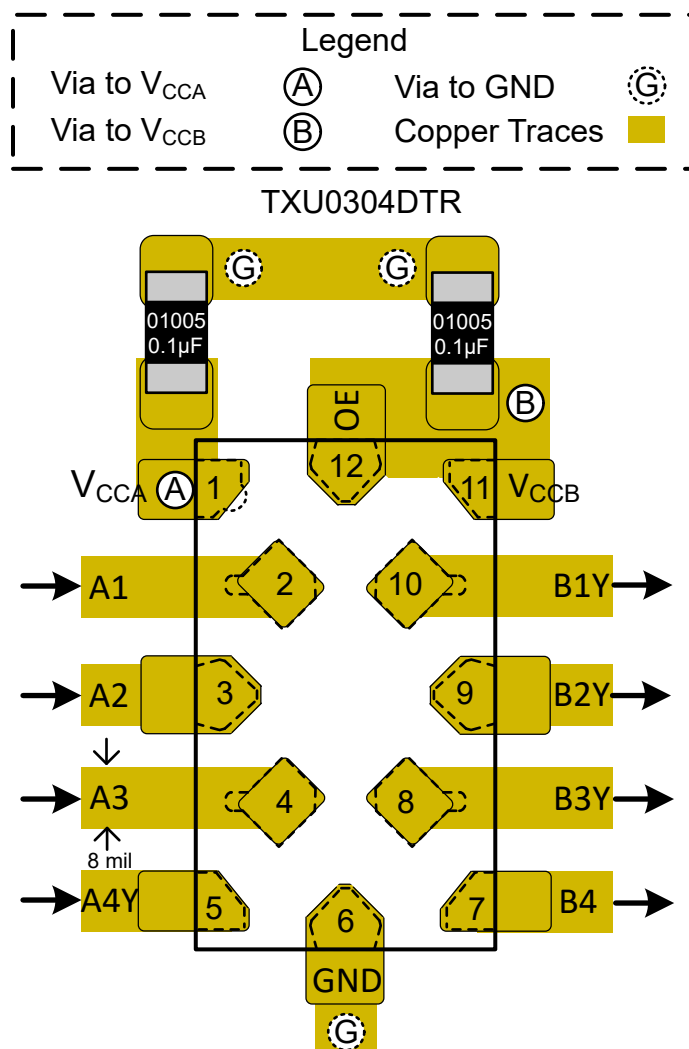
图 12-1. 布局示例 - TXU0304
