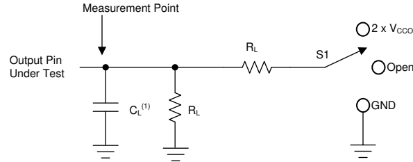
图 8-1. 负载电路
