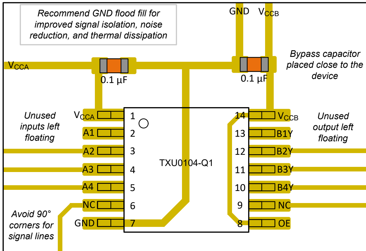
图 12-1. Layout Example - TXU0104-Q1
