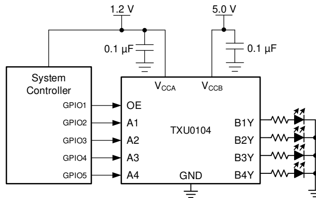
图 8-1. TXU0104 LED 驱动器应用
