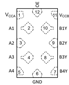
图 4-4. DTR 封装 12 引脚 X2SON 透明俯视图
