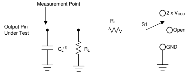
图 6-1. 负载电路
