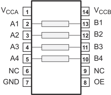
图 4-2. PW 封装，14 引脚 TSSOP（顶视图）
