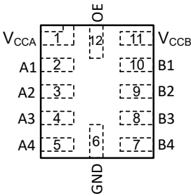
图 4-4. RUT 封装，12 引脚 UQFN (透明顶视图)
