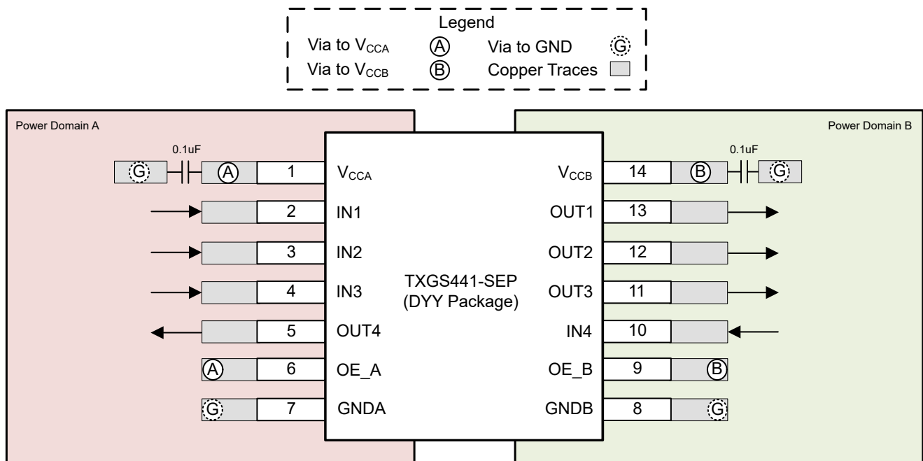
图 8-3. 布局示例
