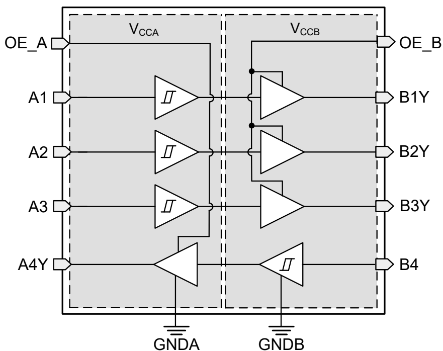
功能方框图
