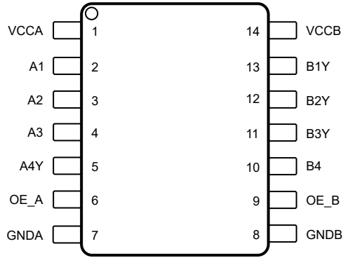
图 4-1. TXGS441-SEP DYY 14 引脚 SOT 顶视图
