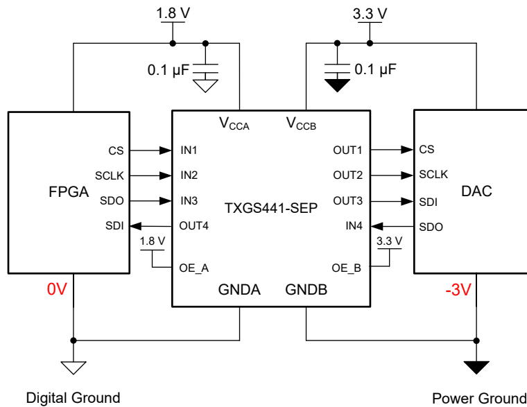
图 8-1. 航天应用中的 TXGS441-SEP
