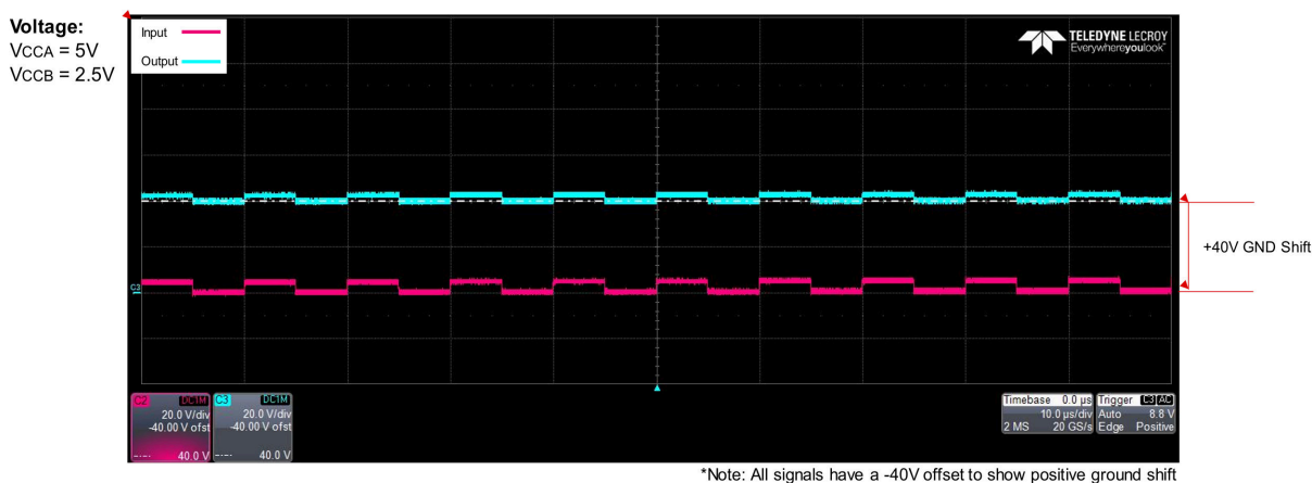
图 8-2. 显示了 5V 至 2.5V I/O 转换的 -40V (顶部) 和 +40V (底部) 接地漂移的波形
