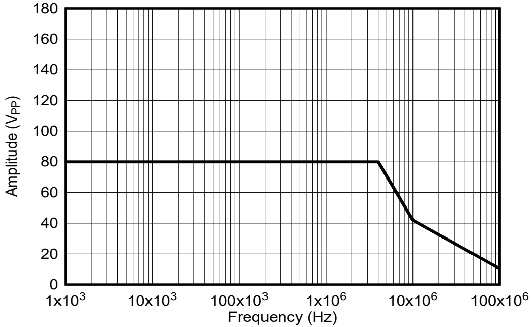
图 7-3. 交流噪声抑制图
