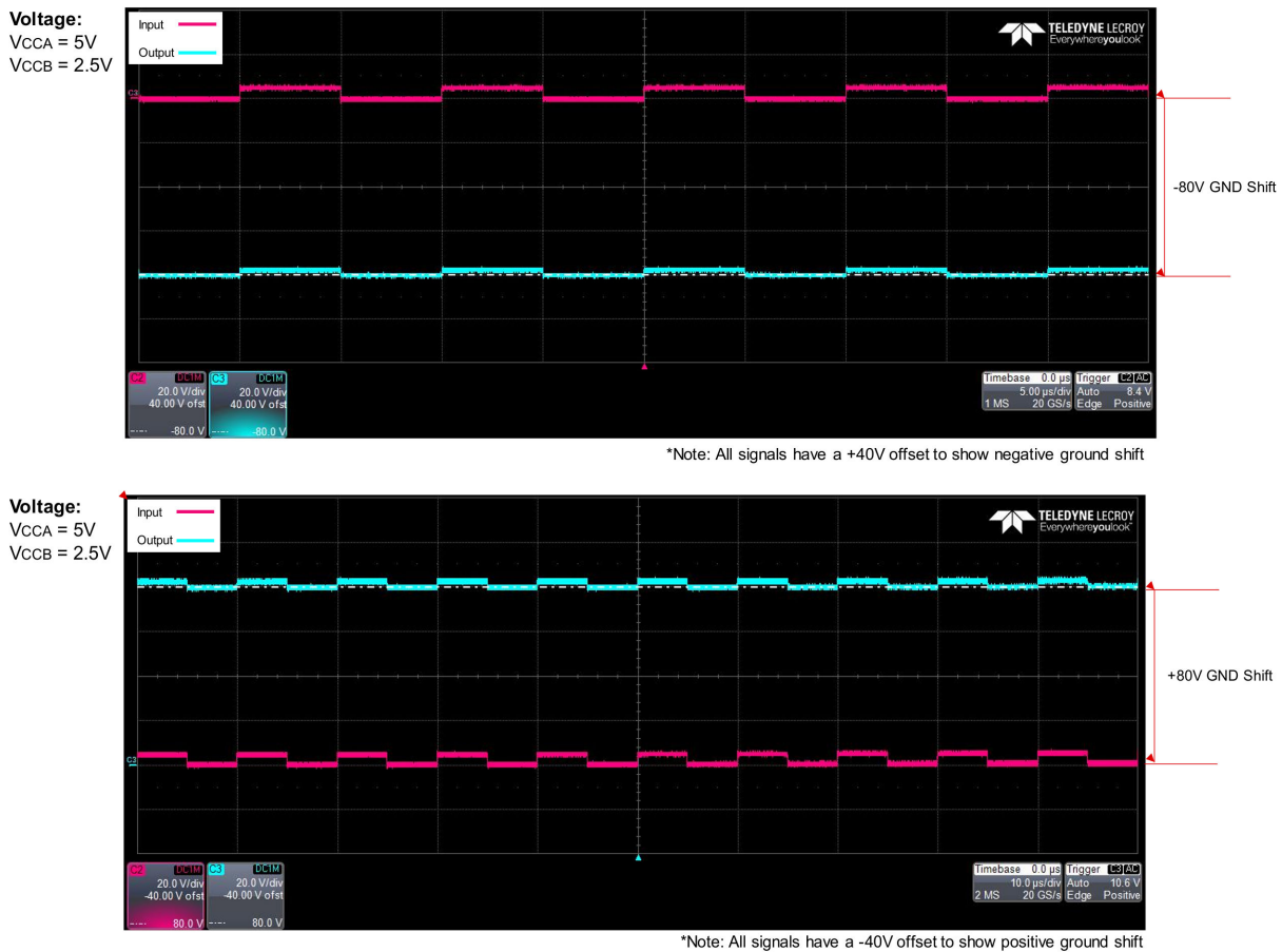
图 8-2. 显示了 5V 至 2.5V I/O 转换的 -80V ( 顶部 ) 和 +80V ( 底部 ) 接地漂移的波形
