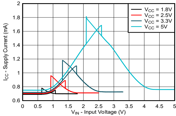
图 5-3. 电源电流 ( I_{CC} ) 与输入电压 ( V_{IN} ) [TXG0x041] 间的关系
