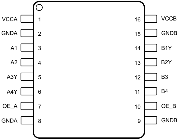
图 4-4. TXGx042DBQ 16 引脚 QSOP 顶视图
