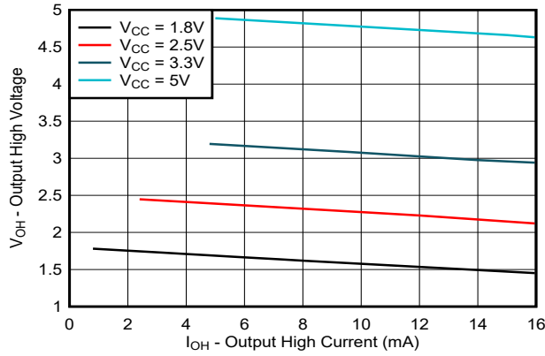
图 5-1. 输出高电压 ( V_{OH} ) 与源电流 ( I_{OH} ) 间的关系
