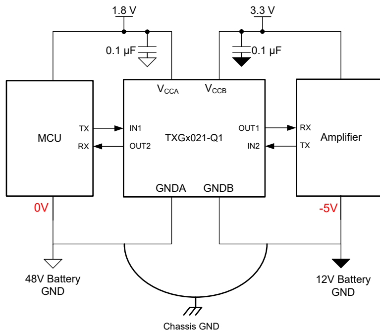
图 8-1. 汽车中的 TXG8021-Q1
