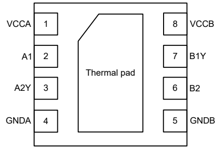
图 4-1. TXGx021DSG 封装 8 引脚 WSON ( 顶视图 )
