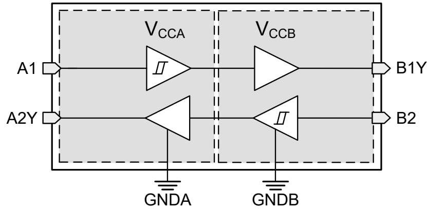
图 7-1. TXG8021-Q1 功能方框图
