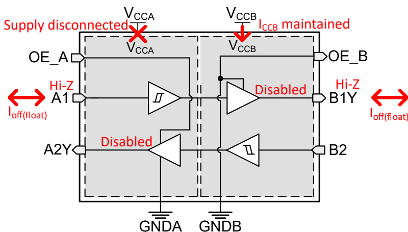
图 7-2. V_{CC} 断开特性
