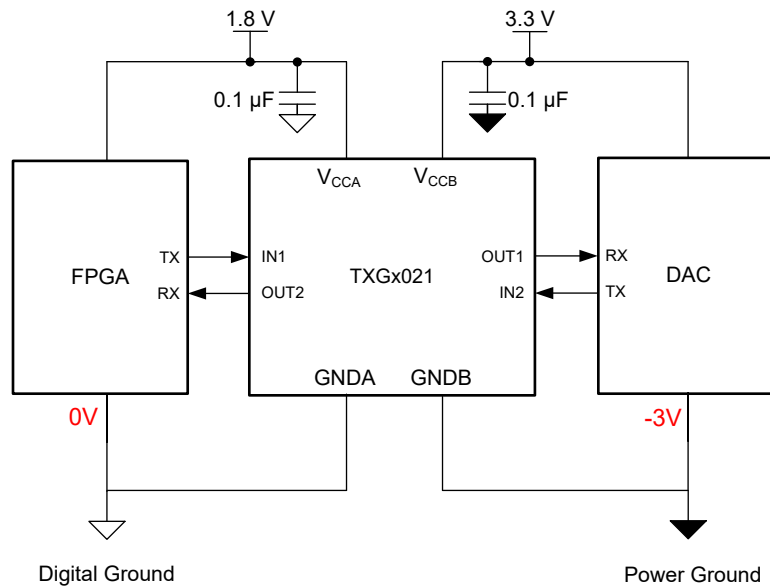
图 8-1. 测试和测量中的 TXG8021
