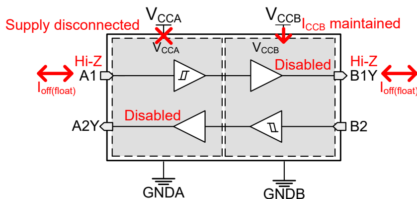
图 7-2. V_{CC} 断开特性
