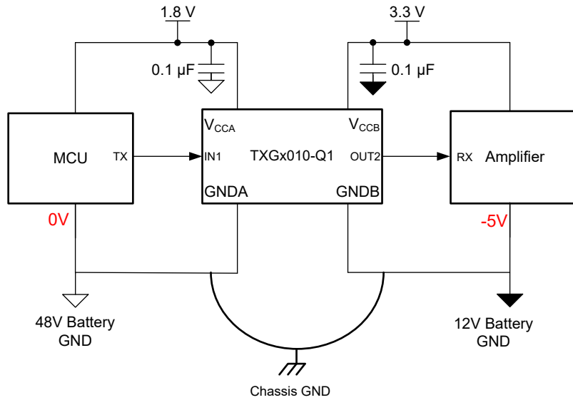
图 8-1. 汽车中的 TXG8010-Q1
