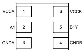
图 4-1. TXGx010DSE 封装 6 引脚 WSON ( 顶视图 )
