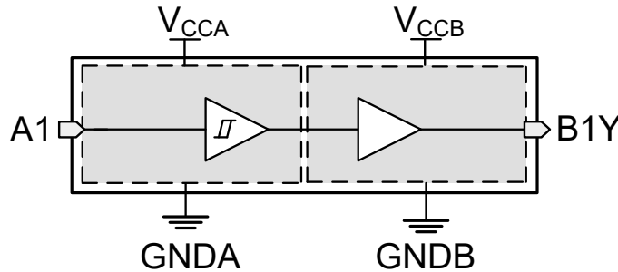
图 7-1. TXG8010-Q1 功能方框图
