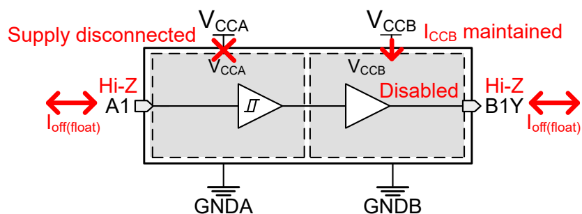
图 7-2. V_{CC} 断开特性
