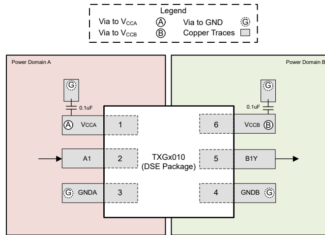
图 8-3. D 布局示例
