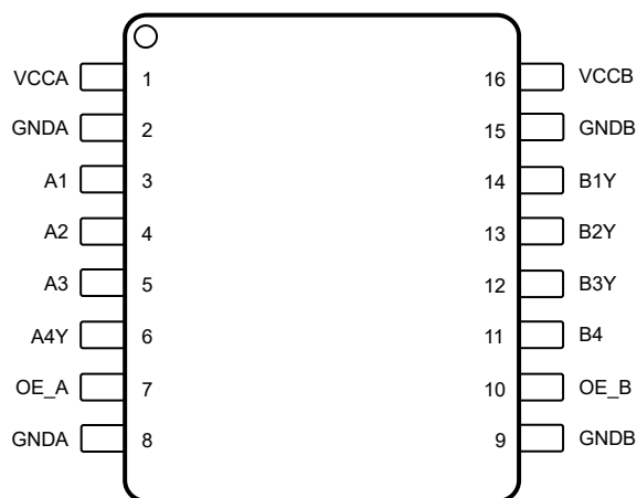
图 4-5. TXG4041 DBQ 16 引脚 QSOP 顶视图
