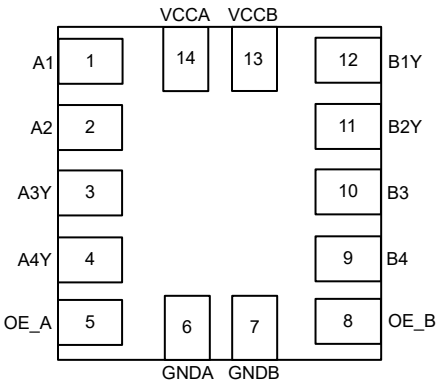
图 4-2. TXG4042 RUC 封装 14 引脚 X2QFN 顶视图
