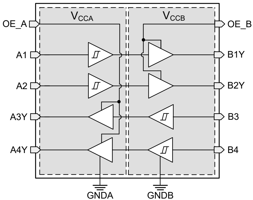
图 7-2. TXG4042 功能方框图
